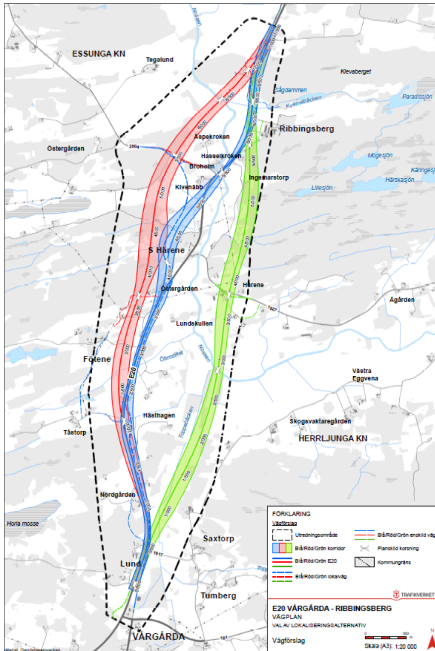
Figur 1. Utredningsområde och föreslagna vägkorridorer.
