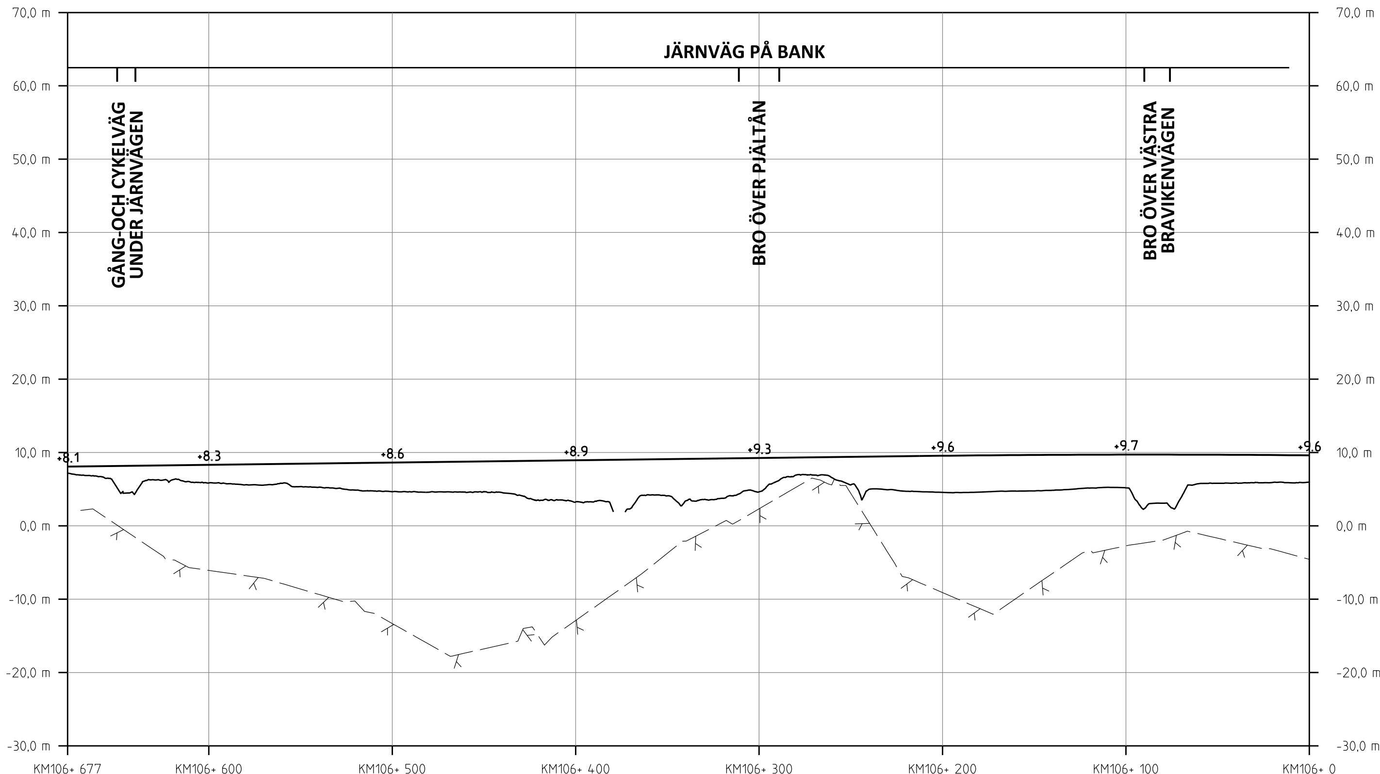
PROFIL SPÅRPROFIL LÄNGS NEDSPÅRET (ÖSTLIGA SPÅRET)
