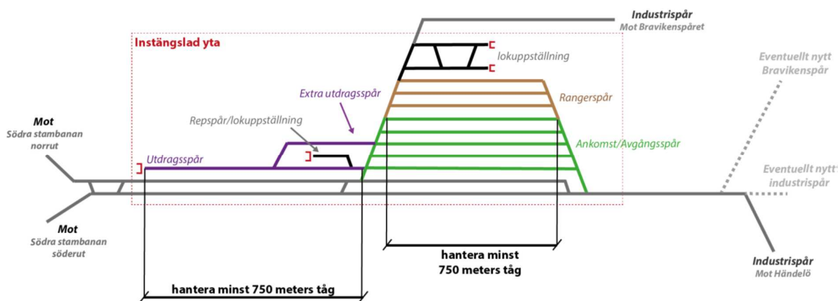
Figur 17. Funktionsskiss över Norrköpings bangård i UA2
