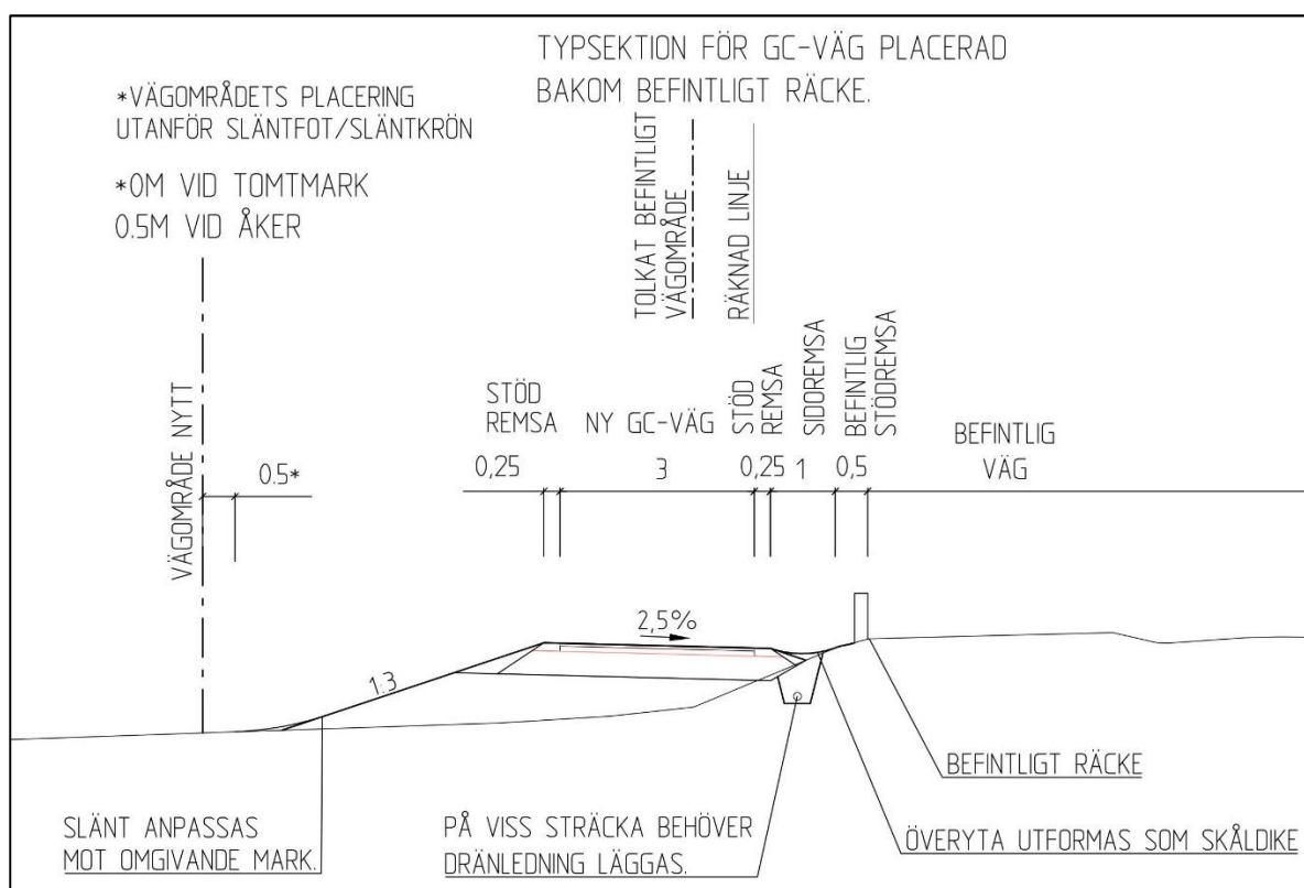
Figur 10. Typsektion 3. Lösning för trånga sektioner med 1 m bred grusbelagd sidoremsa och befintligt räcke inom sidoremsan.
