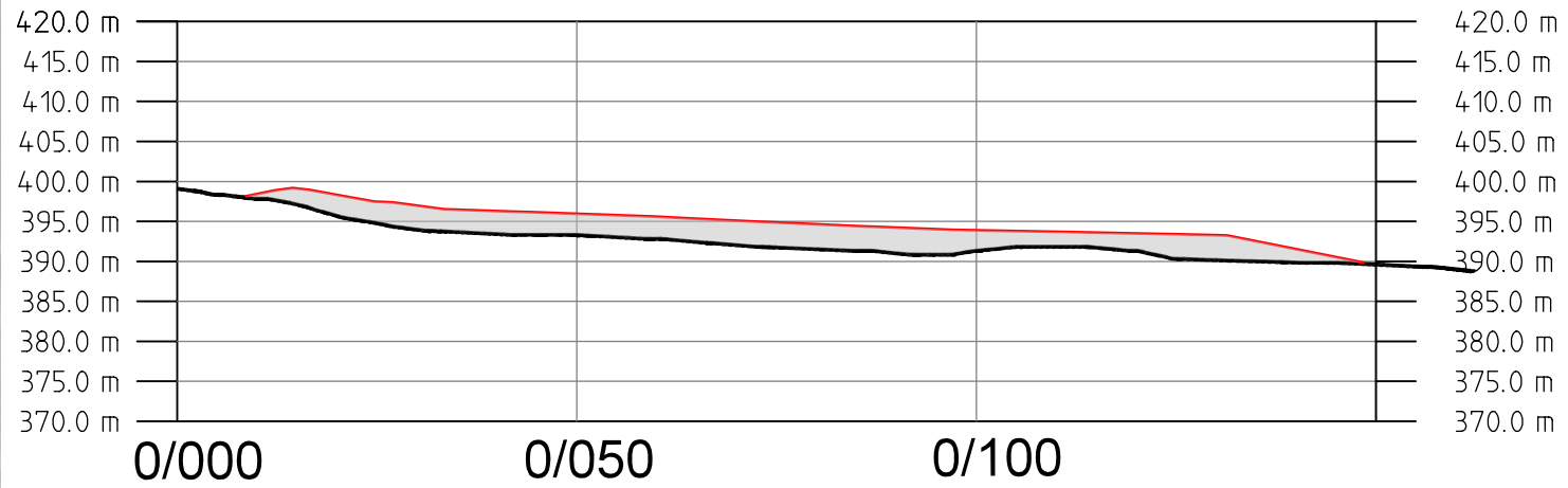
Längdprofil
