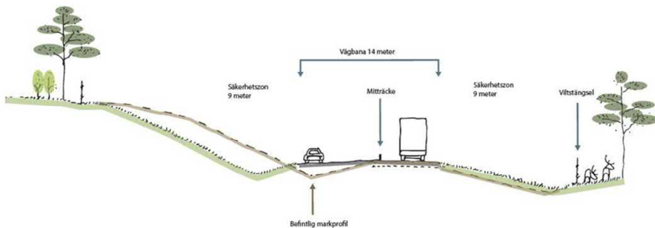
Figur 11. Illustration över 2+1 väg, där E10 breddas till 14 m med mitträcke och viltstängsel och 9 m säkerhetszon.
