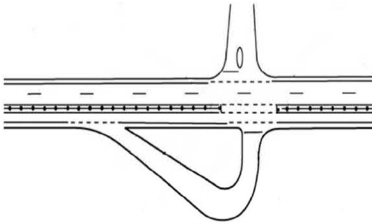
Figur 13. Principskiss av korsningstyp ögla.
