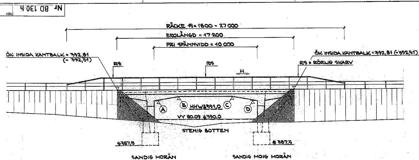
ELEVATION 1:100
