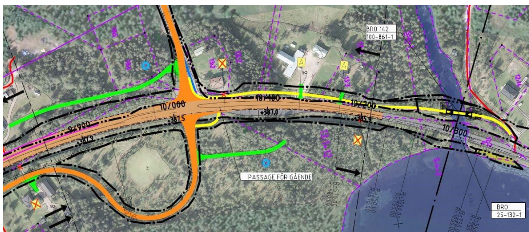
Figur 23. C-korsning i söder om Skaulo där avbrott för viltstängsel och mittenräcke görs genom Skaulo. Placering av gång- och cykelväg syns till höger i bild, gång- och cykelbro kopplas ihop med befintlig gång- och cykelväg norrut.
