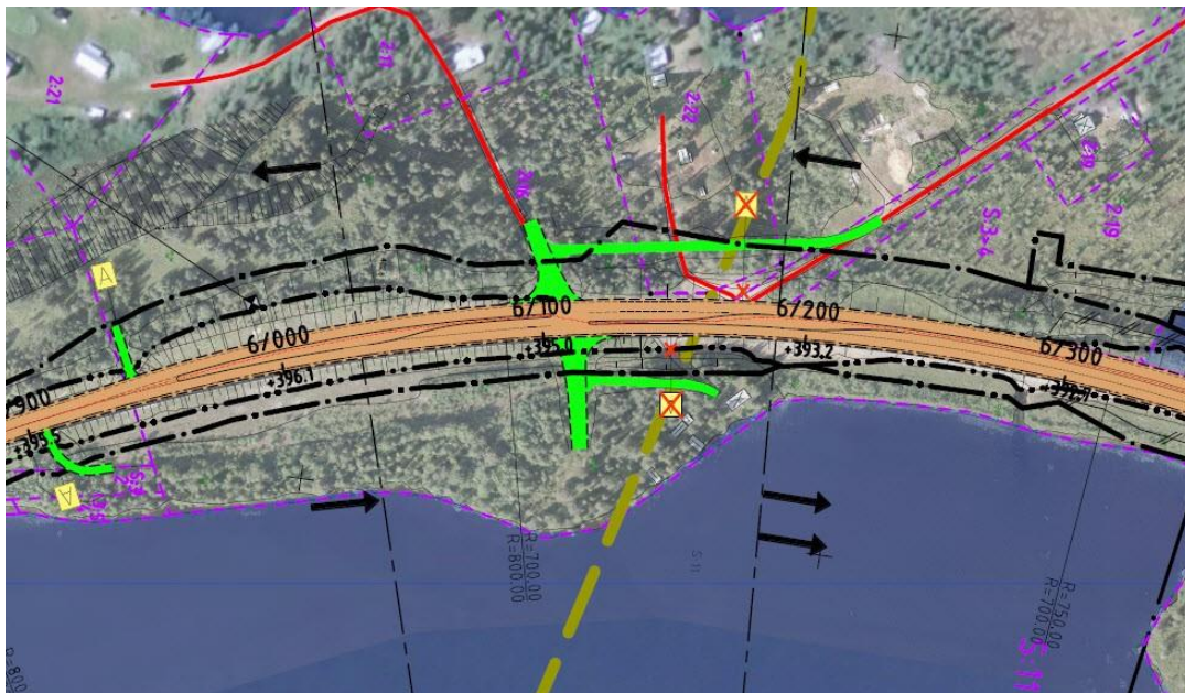
Figur 21. Ny korsning i Moskojärvi vid km 6/100 som ligger utmed Kenttjärvi med föreslagna placeringar av nya enskilda vägar.
