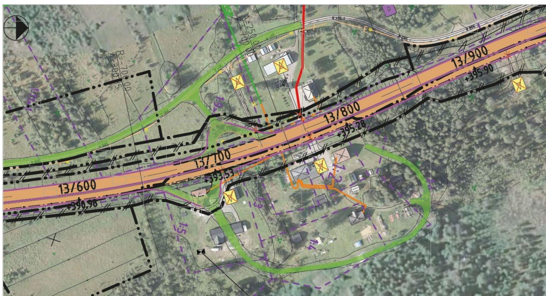
Figur 16. Ögla i Alapää, söder om Puoltikasvaara, ny enskild väg föreslås på den östra sidan till fastigheter som i dagsläget har direktutfarer mot E10. På den västra sidan föreslås en justering av befintlig gång- och cykelväg mellan Skaulo och Puoltikasvaara.
