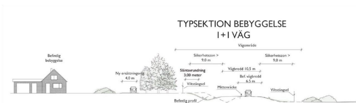
Figur 15. Typsektion från områden med bebyggelse där E10 anläggs som 1+1 väg med en vägbredd på 10,5 meter.
