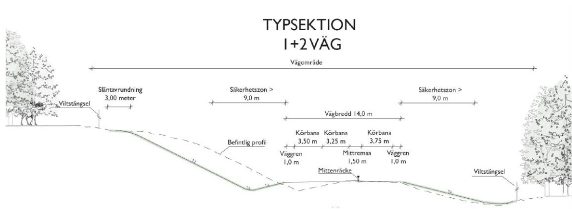
Figur 8. Typsektion över nytt vägrum med 1+2 väg.
