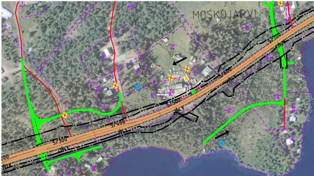
Figur 20. Nya korsningar i Moskojärvi vid km 5/300 och 5/700 som ligger utmed Kenttjärvi med föreslagna placeringar av nya enskilda vägar.
