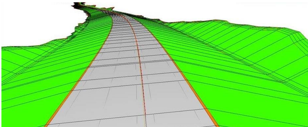
Figur 9. Utsnitt över ny vägbreddning med ny släntutformning med innersläntlutning på 1:4. Vägbreddning medför att vägområde utökas med mellan 4 till 8 meter.
