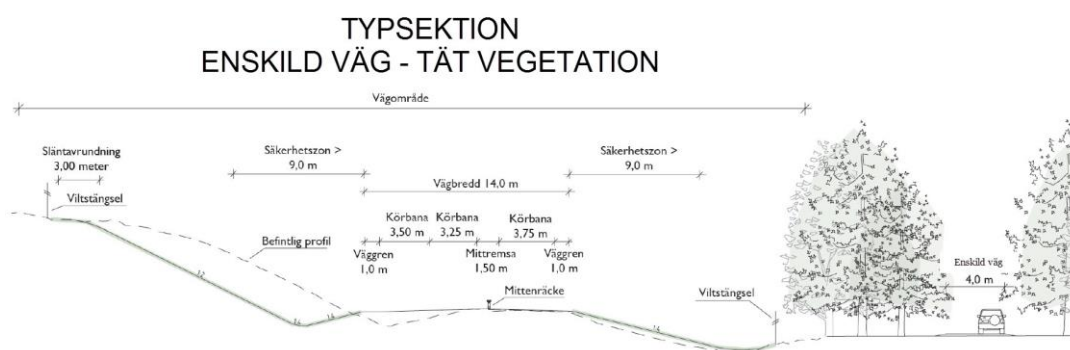
Figur 10. Typsektion för att illustrera placering av ny enskild väg där tät skogsvegetation växer i anslutning till E10 med syfte att minimera vägrummets utbredning.
