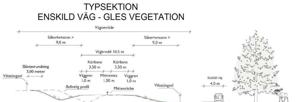
Figur 11. Typsektion för att illustrera principen av placering av ny enskild väg när sidoområdena utgörs av gles vegetation.
