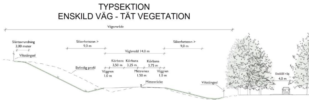
Figur 10. Typsektion för att illustrera placering av ny enskild väg där tät skogsvegetation växer i anslutning till E10 med syfte att minimera väggrummets utbredning.
