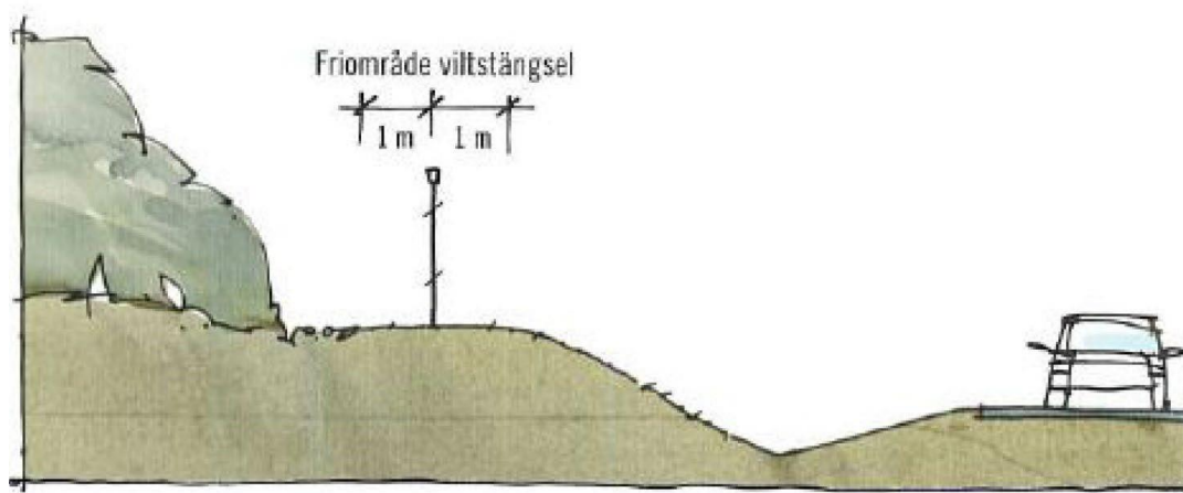
Figur 34. Principskiss över placering av viltstängsel från Vägen. En bok om vägarkitektur (Vägverket, 2006)
