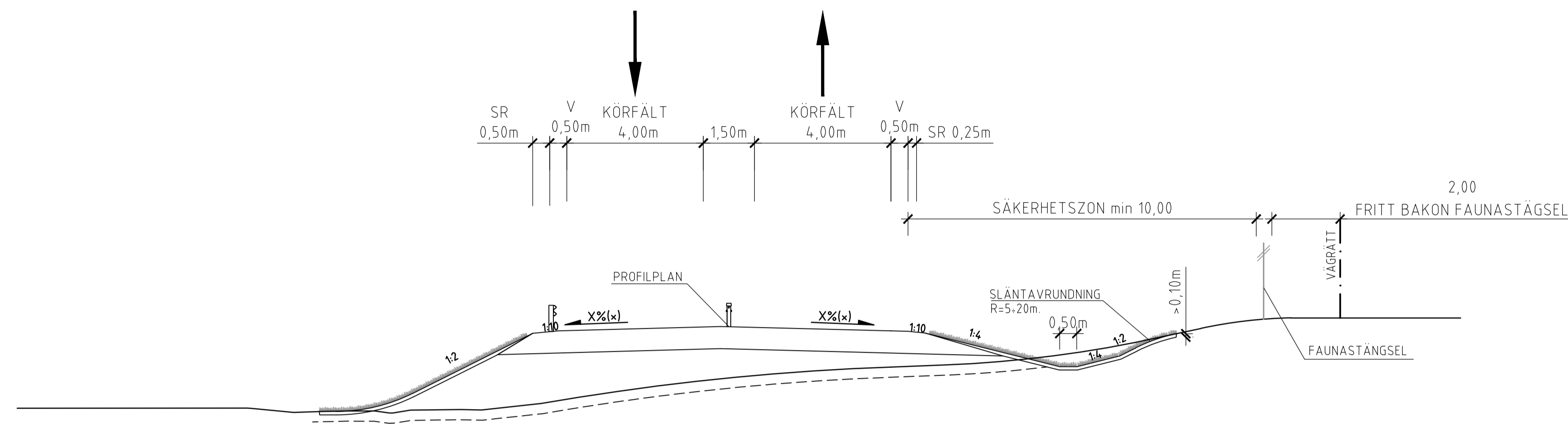
MÖTESFRI VÄG (1+1). SKÄRNING OCH BANK SKALA 1:100
