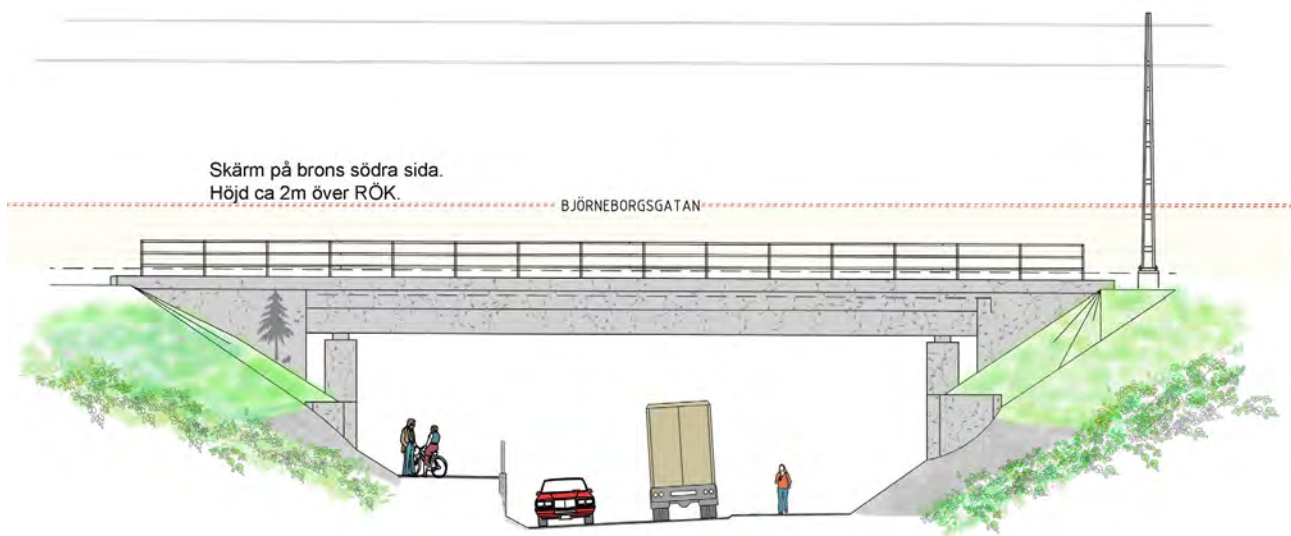
Figur 4.2:7 Broskiss, ny dubbelspårig järnvägsbro vid E14/Björneborgsgatan.
