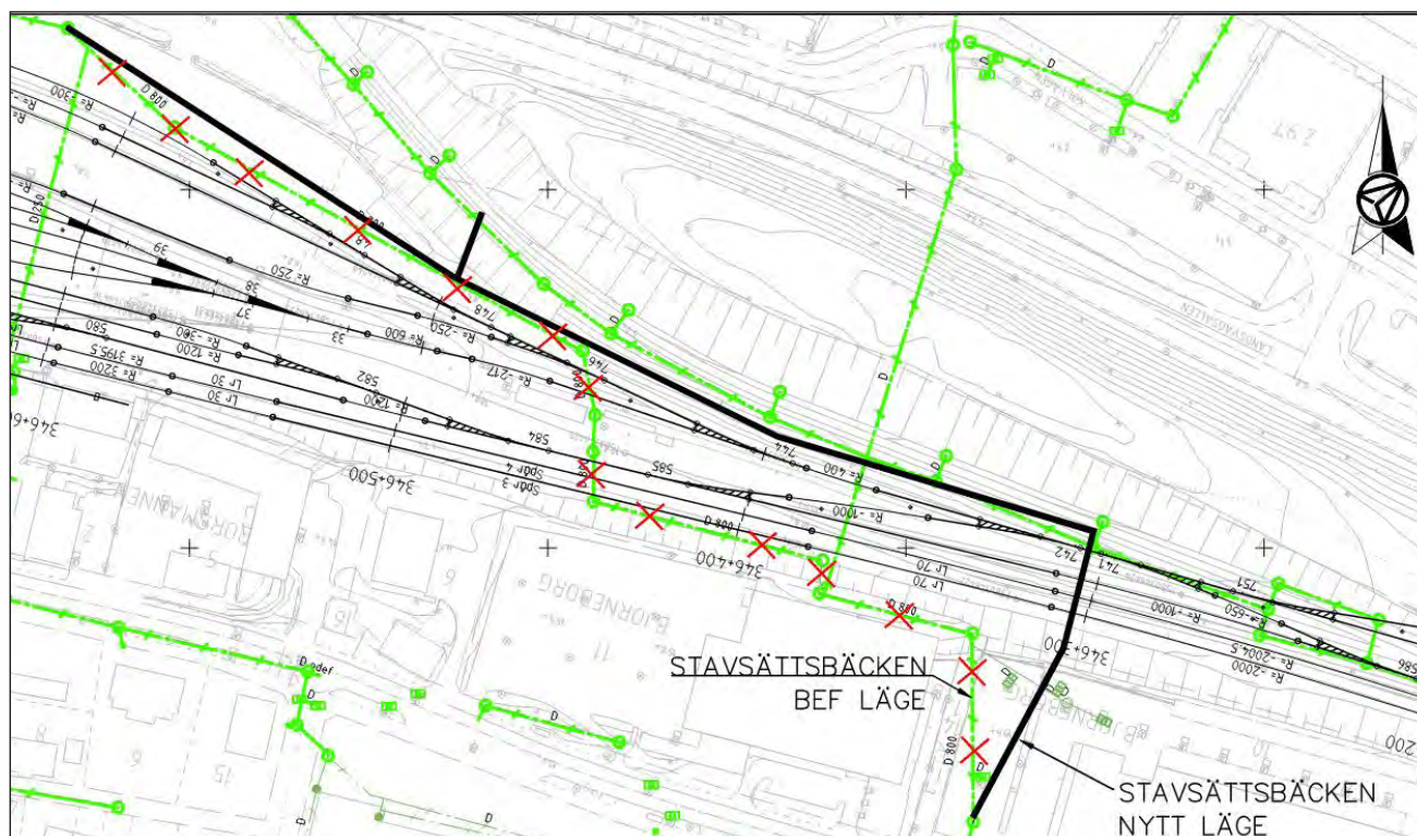
Figur 4.2:2 Föreslagen omläggning av dagvattenkulvert för Stavsättsbäcken (markerad i svart). Spårmodellen är redovisas i tunna svarta linjer och befintligt dagvattensystem i grönt. Röda kryss är rivningskryss.
