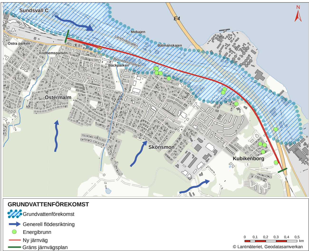
Figur 3.5:9 Karta över grundvattenmagasinet tillsammans med planerad järnväg samt energibrunnar belägna inom 100 meter från planerad järnväg. Översiktligt flödesmönster visas med blå pilar.
