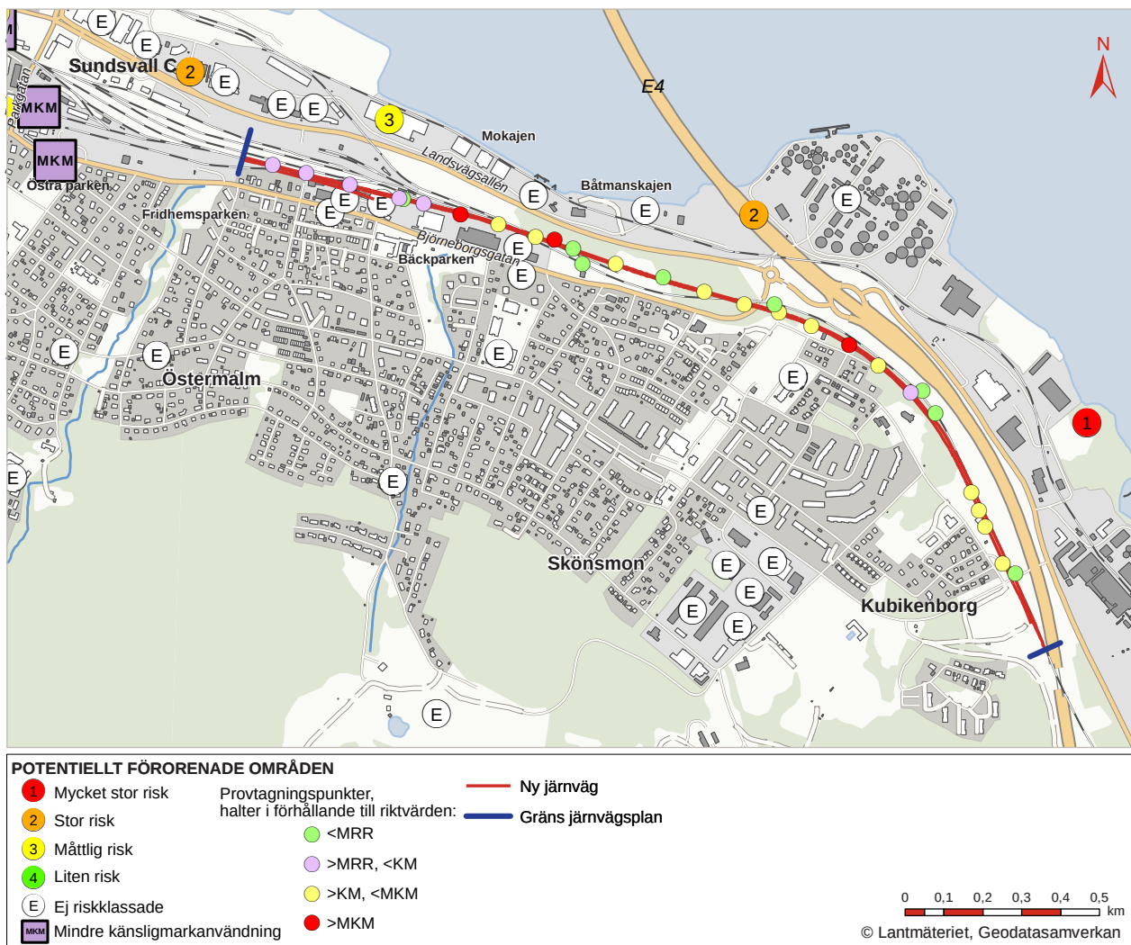
Figur 3.7:3 Potentiellt förorenade områden i planområdets närhet samt uppmätta halter från genomförda undersökningar i förhållande till riktvärden. Objekt riskklassade (1-4) enligt Naturvårdverkets metodik för inventering av förorenade områden. Riskklass 1 innebär att verksamheten utgör en mycket stor risk för oönskade effekter på människors hälsa och miljön, riskklass 2 utgör stor risk, riskklass 3 utgör måttlig risk och riskklass 4 utgör liten risk. Objekt som inte är riskklassade är markerade med ett E. Objekt markerade med "MKM" avser objekt som redan är efterbehandlade till nivån mindre känslig markanvändning.
