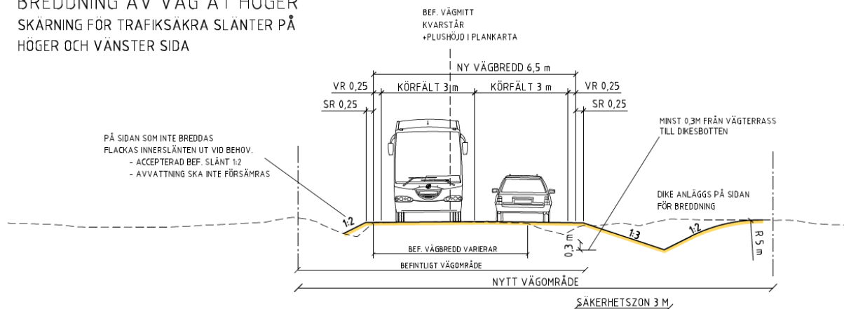
Figur 25 Typsektion i jordskäring
