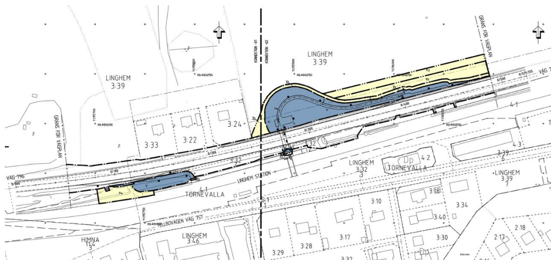
Figur 20. Utdrag ur vägplanens plankartor väg 796 Linghem station, nytt hållplatsläge
