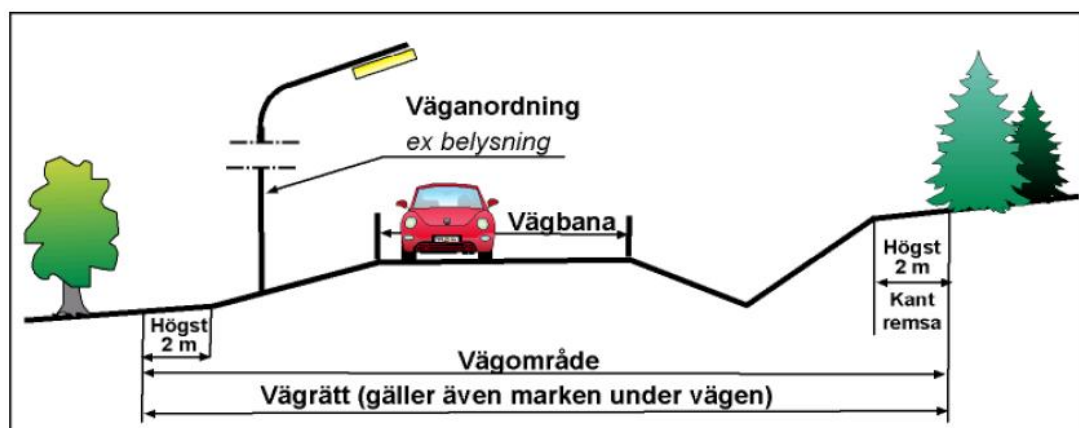
Figur 34. Vägområde med kantremsor. Figuren illustrerar en väg men samma princip gäller för gång- och cykelvägen.
