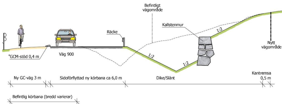
Figur 33. Sektion med kallstenmur öster om väg 900 mitt emot Rörviks camping.
