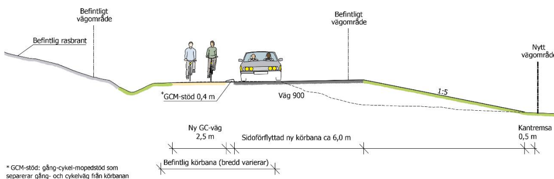
Figur 35. Sektion vid sidoförflyttning av väg 900 förbi rasbrant söder om Hamburgsund.
