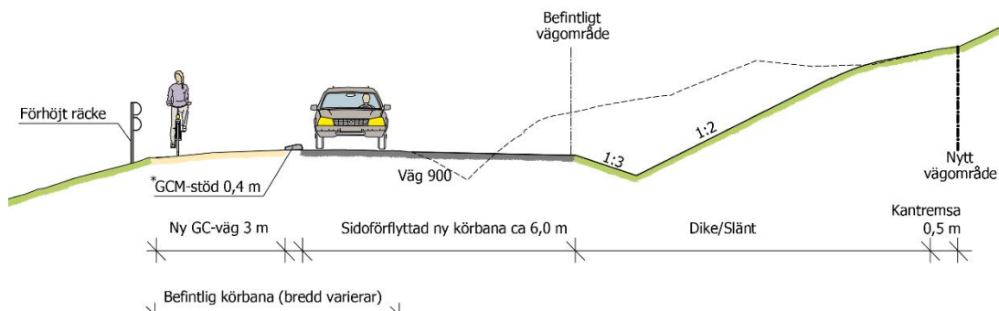
Figur 32. Sektion vid sidoflyttning av väg 900 förbi Rörviks camping.
