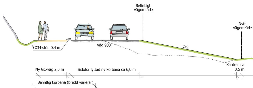
Figur 31. Sektion vid sidoförflyttning av väg 900 intill befintlig bergsslänt norr om Slottet.
