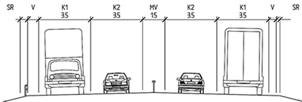
Figur 22. Illustration av ny sektion och mittremsa. Med vägrenar på 0,5 m bredd blir den totala belagda ytan 16,5 m.
