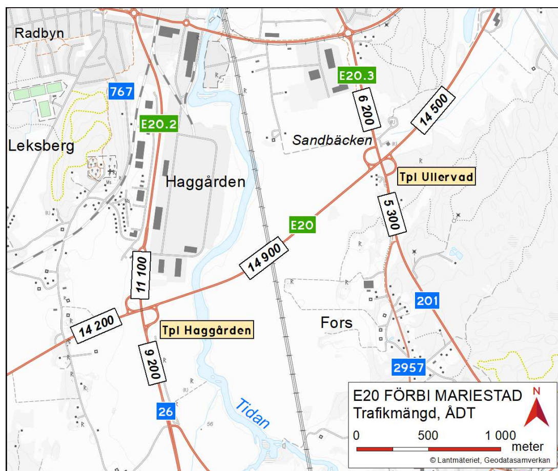
Figur 10. Trafikmängder år 2045 för Nollalternativet.
