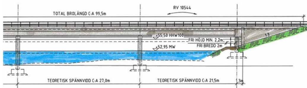
Figur 26. Dela av ny bro över Tidan.
