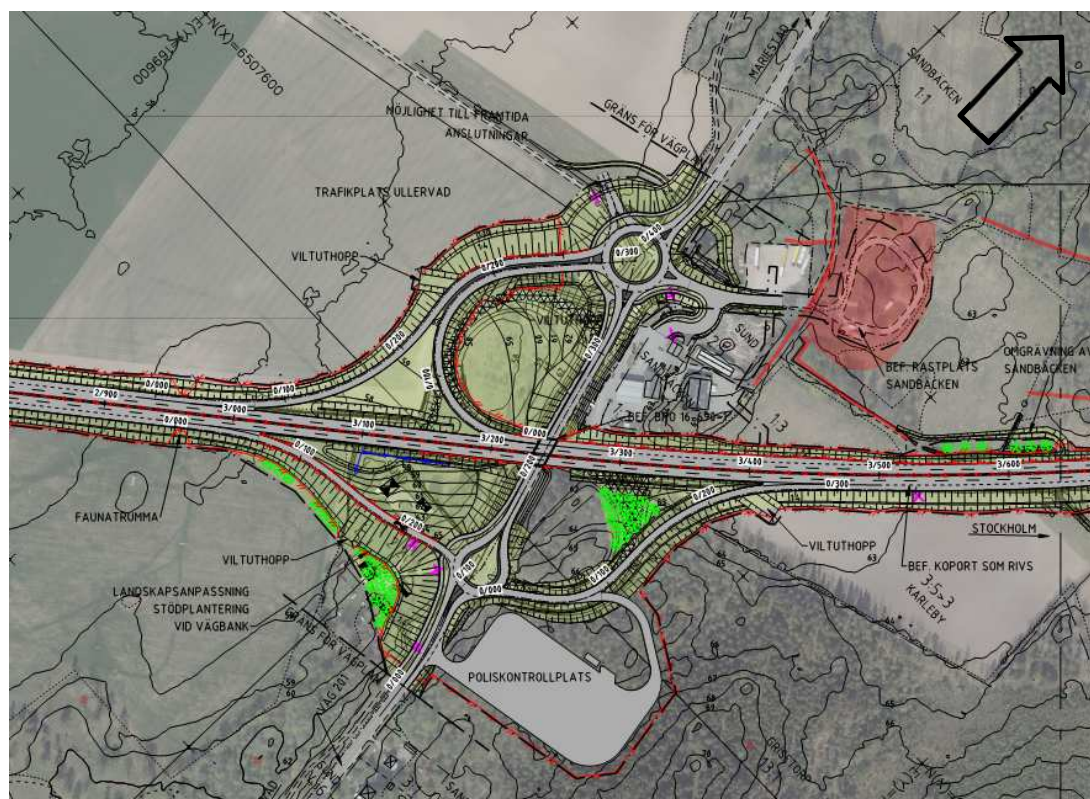
Figur 24. Trafikplats Ullervad efter föreslagen ombyggnation. E20 går här i nordöstlig riktning vilket medför att den övre sidan i bilden ligger på den västra sidan av E20.
