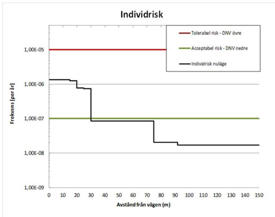
Figur 15. Individrisknivå för nuläget. Acceptabel risk erhålls på 30 meter ifrån väg E20.
