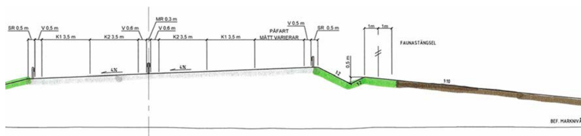
Figur 28. Typsektion för E20 öster om Tidan med brukbar slänt.
