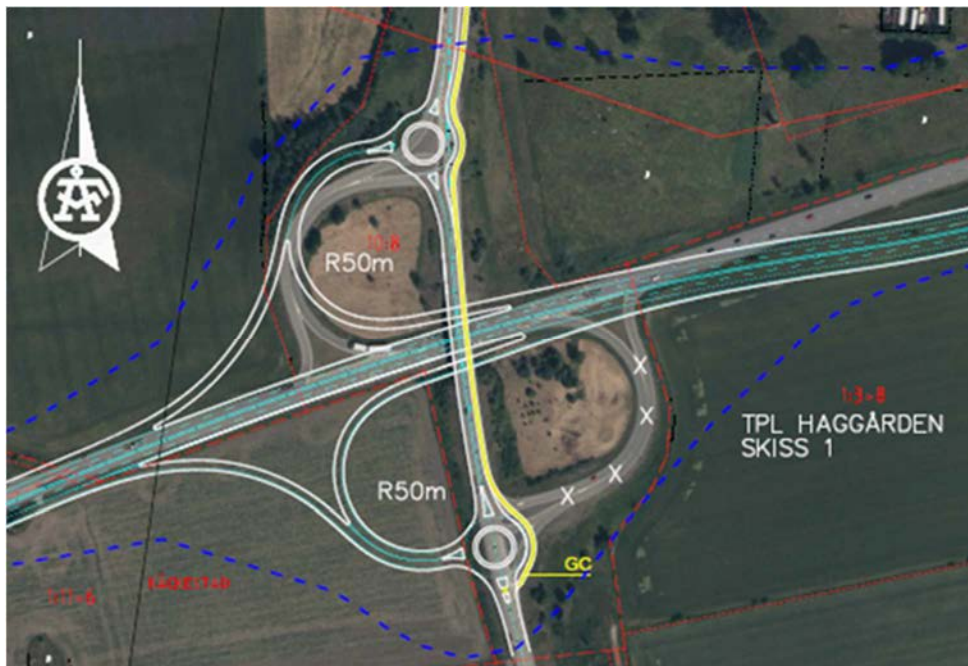
Figur 29. Klöverutformning (båda klöverbladen på västra sidan).
