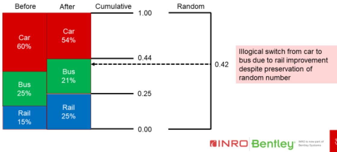
Figur 18. Illustration av valprocessen vid Monte-Carlo simulering. Källa: Bentley.
