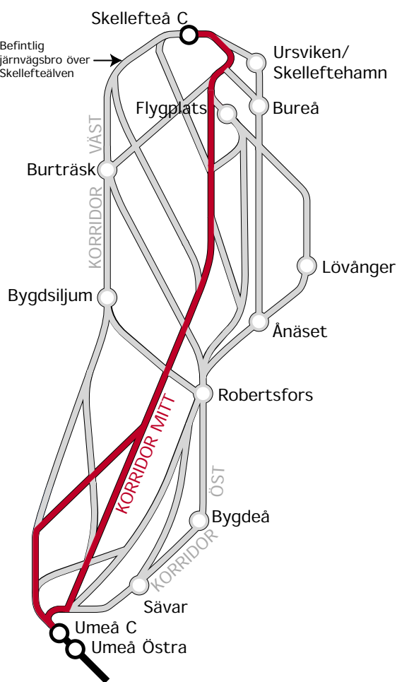
Figur 7.10:2 Bortsorterat alternativ - korridor Mitt i sin helhet.
