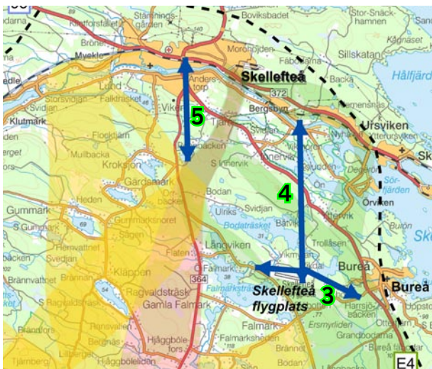
Figur 7.10:4 Bortsorterade dragningar inom korridor Öst vid Skellefteå.
