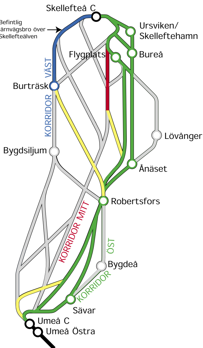
Figur 7.11:1 Illustration av kvarvarande alternativ och kombinationer, se även bilaga 3. Det är dessa alternativ som effekt- och konsekvensbeskrivs i kapitel 8.
