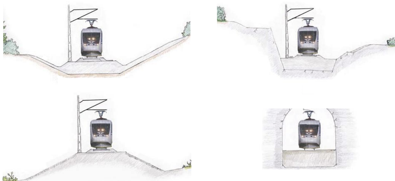
Figur 7.1:1 Principiell uppbyggnad av järnvägen: typsektion i skärning, på bank, i bergskärning samt tunnel.
