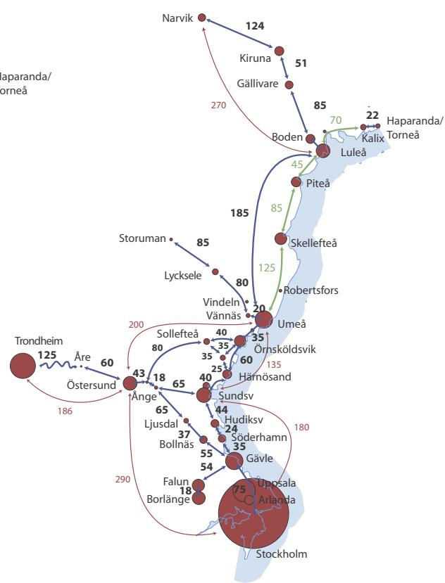
Figur 4.2:4 Restidsavstånd vid ett nollalternativ med Botniabanan utbyggd. Källa: ÅF Infraplan.
