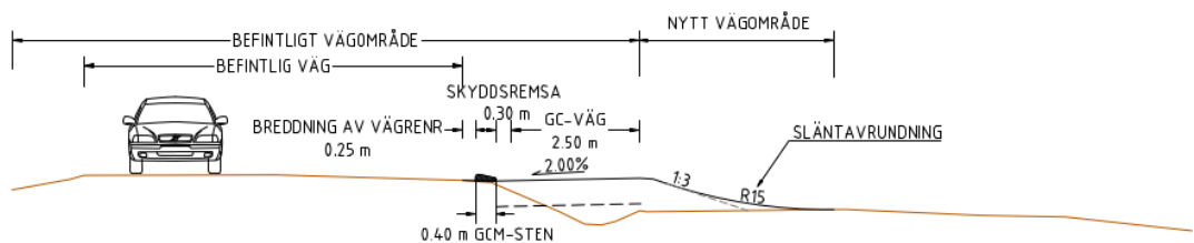
Figur 12 Trång sektion GCM-stöd mot tomtmark
