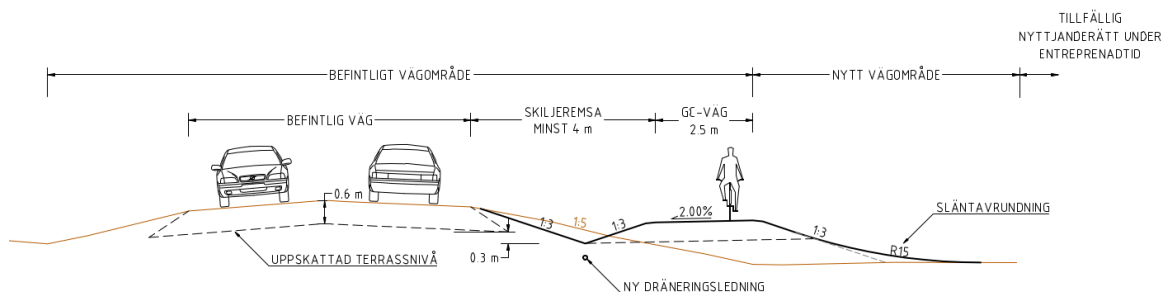
Figur 13 GC-bank anslutning mot slänt vid åkermark och skogsmark med flack innerslänt
