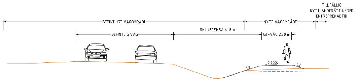
Figur 11 Gång- och cykelväg med skiljeremsa
