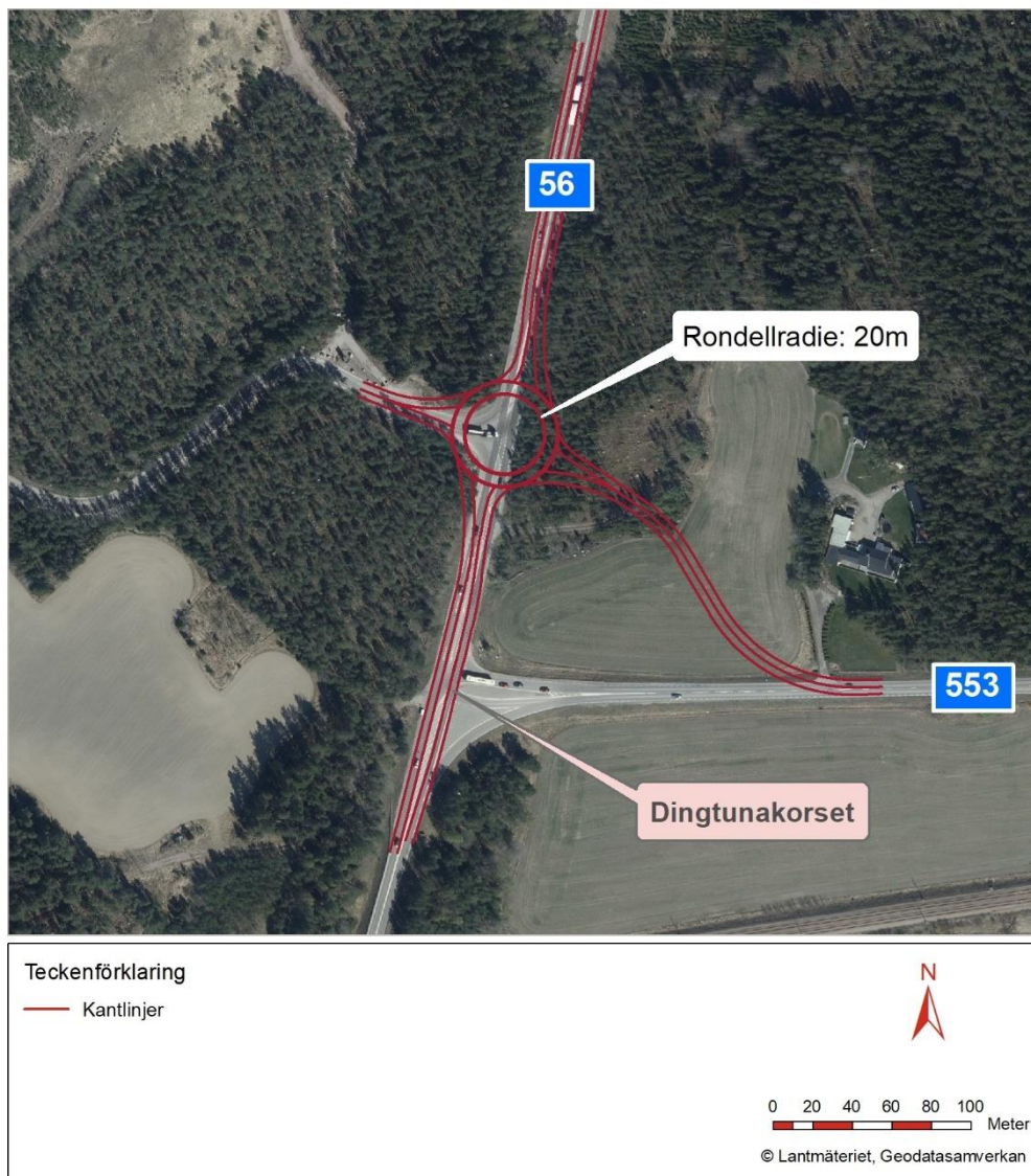
Figur 21. Studerat, bortvalt alternativ med cirkulationsplats.
