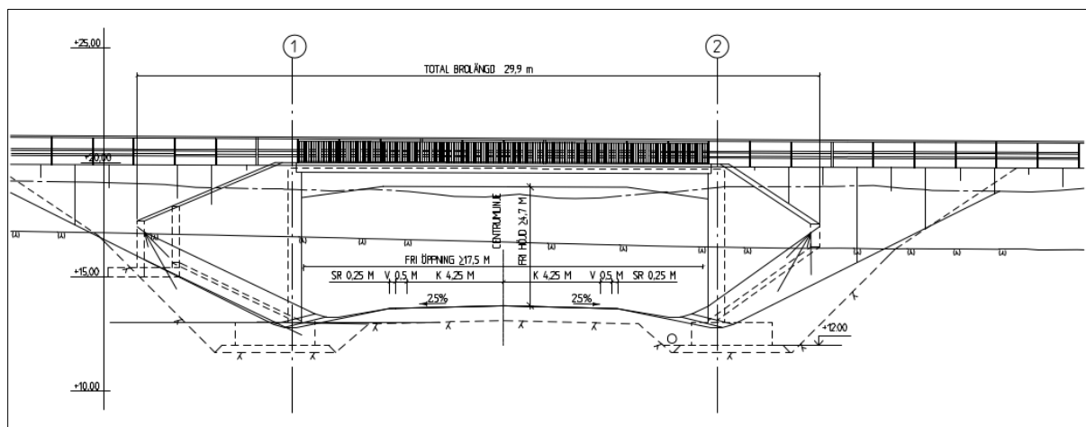
Figur 19. Sektion väg 553 under trafikplatsens bro.
