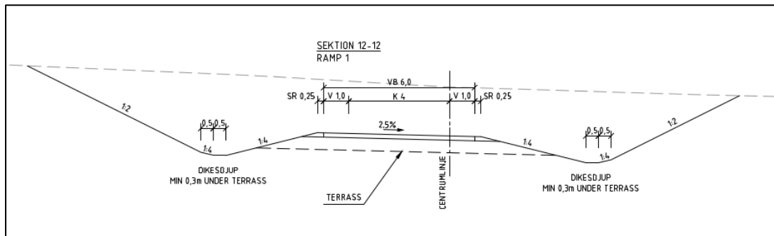
Figur 18. Sektion ramper
