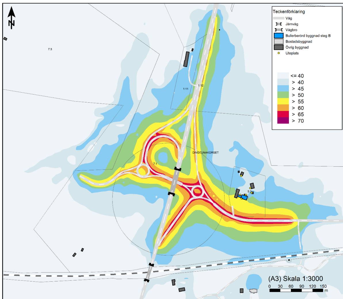
Figur 25. Avgränsningsberäkning, trafik prognosår 2040. Ekvivalent ljudnivå i dBA.
