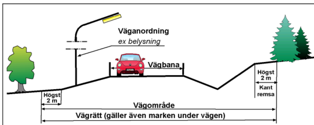
Figur 26. Vägområde med kantremsor.
