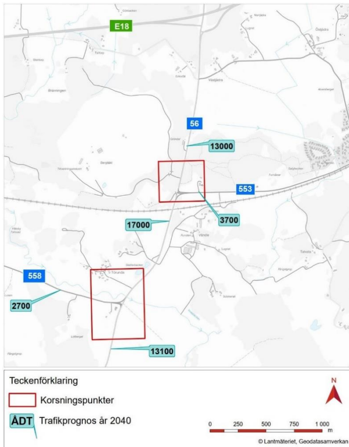
Figur 4. Trafikmängder prognosåret 2040.
