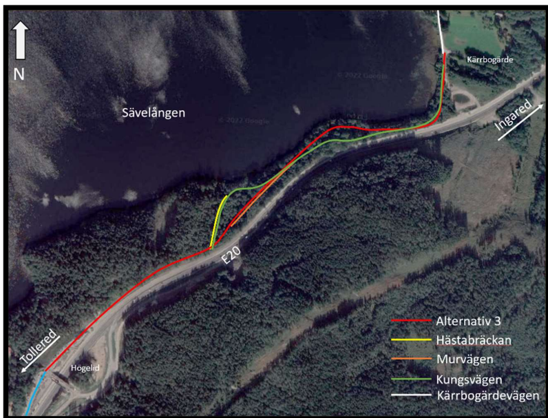
Figur 28. Alternativ 3 - Placering parallellt med murvägen.
