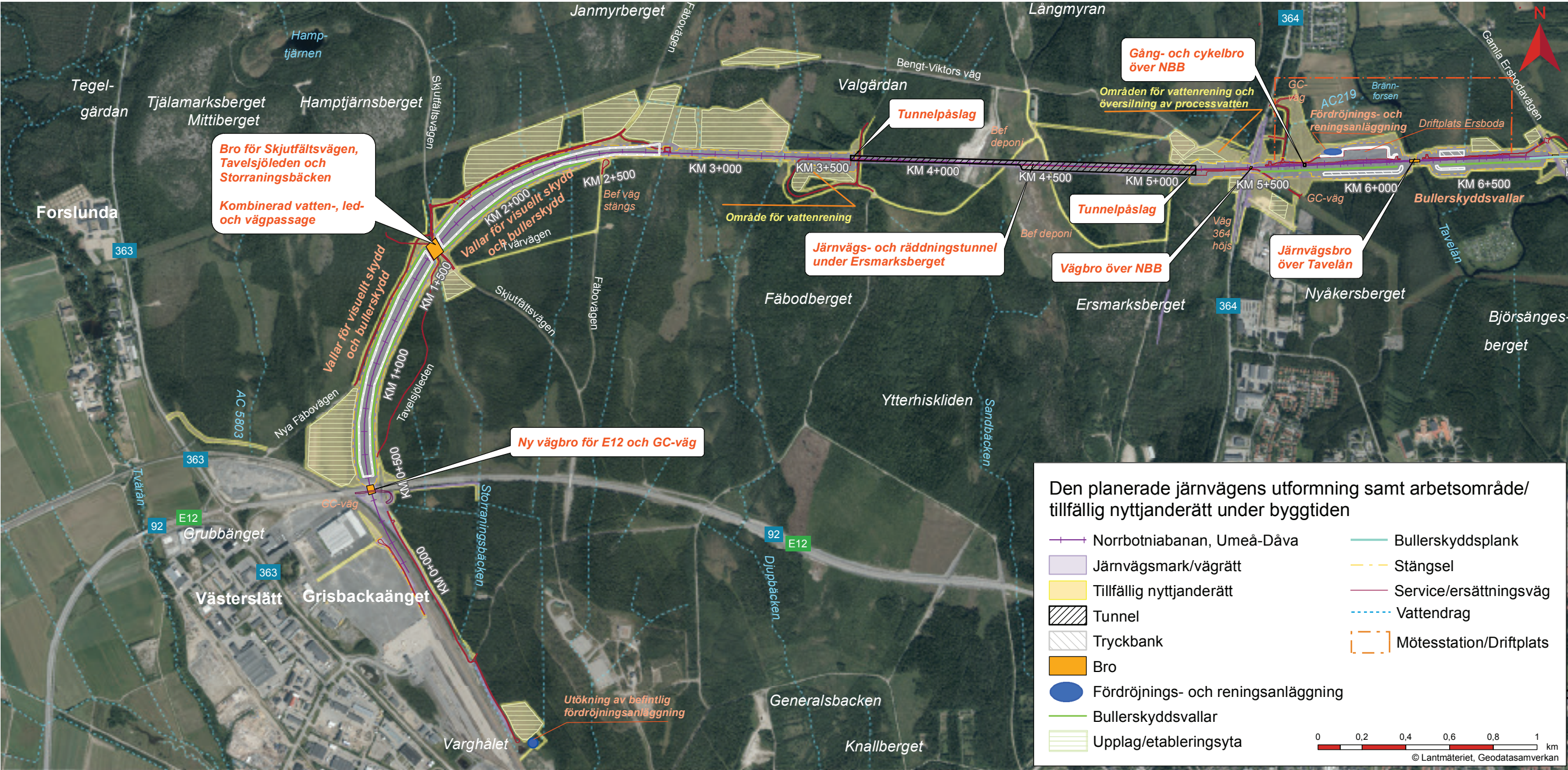
Figur 4.2-11 Den planerade järnvägens utformning samt arbetsområde under byggtiden (område med tillfällig nyttjanderätt).
