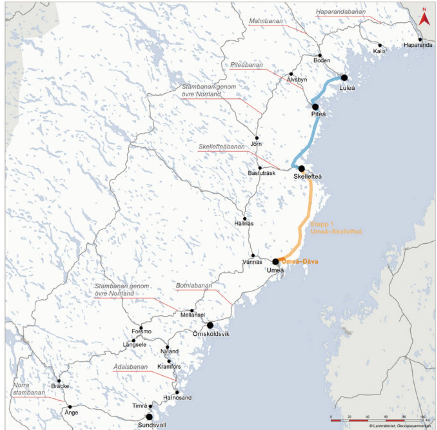
Figur 3.1-1 Befintligt järnvägsnät samt Norrbotniabanan Umeå-Luleå med ettapp 1 Umeå-Skellefteå och sträckan Umeå-Dåva.
