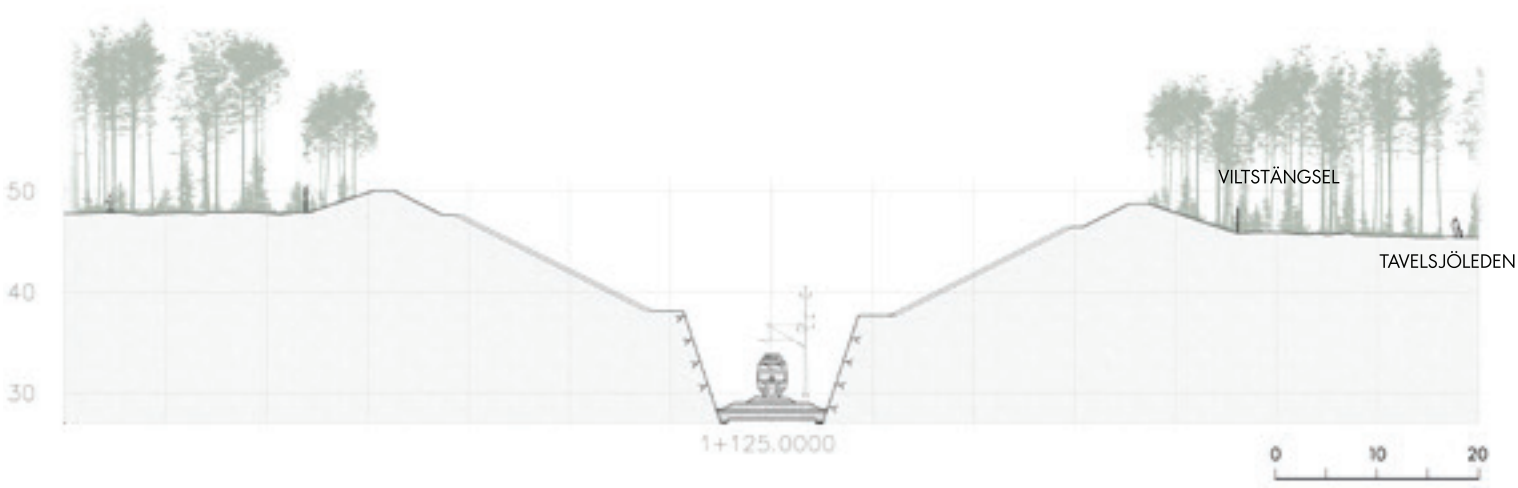
Figur 4.2-3 Skärningen genom I 20-skogen, km ca 1+125.
