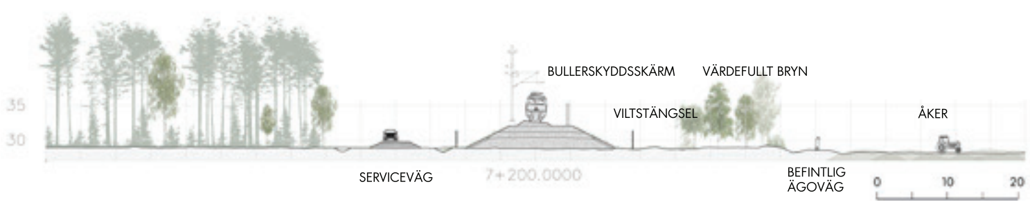
Figur 4.2-4 Järnvägen norr om värdefullt bryn, befintlig bruksväg och det småskaliga mosaiklandskapet vid Tavelån, km ca 7+200.
