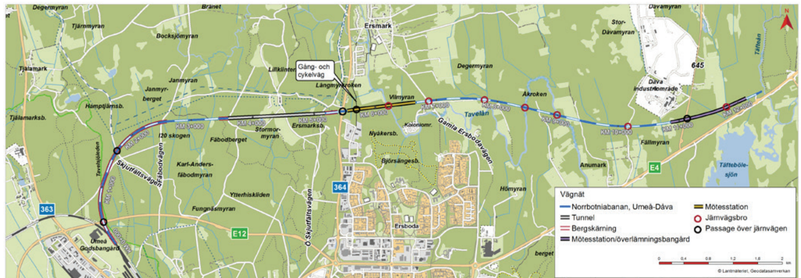
Figur 3.1-2 Befintligt vagnät.
