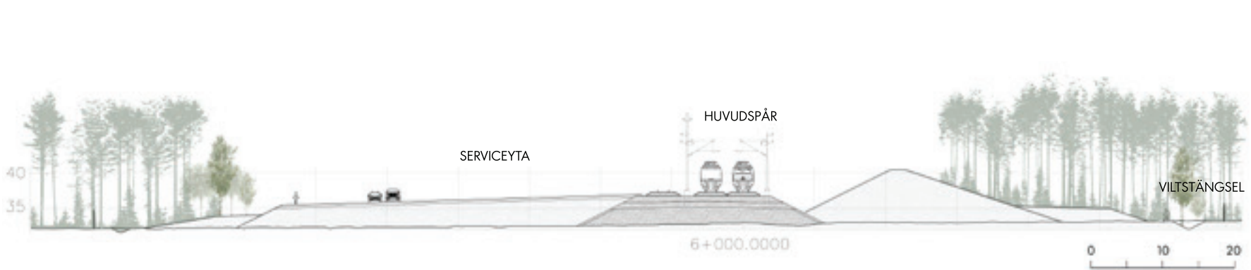
Figur 4.2-5 Järnvägen i anslutning till mötesstationen i Ersboda (Driftplats Ersboda), km ca 6+000.
