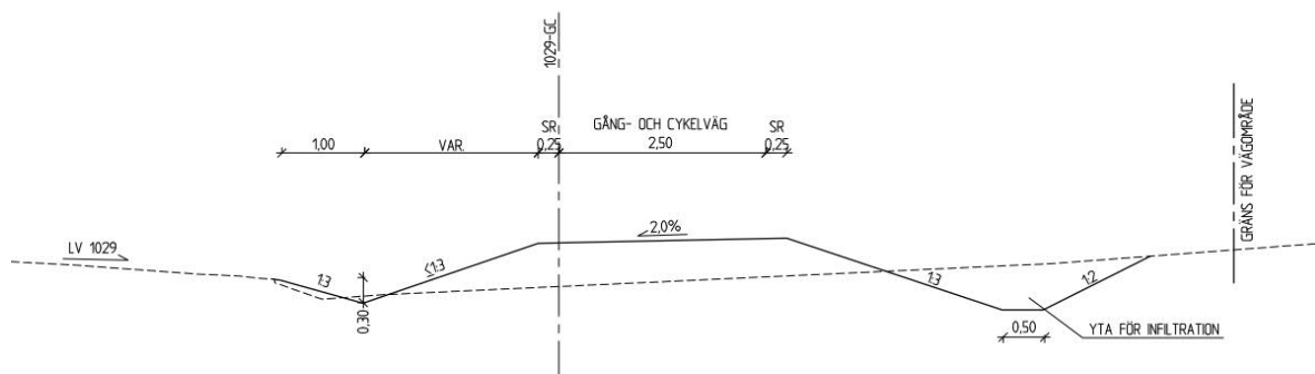
Figur 35. Typsektion fördröjningsdike.
