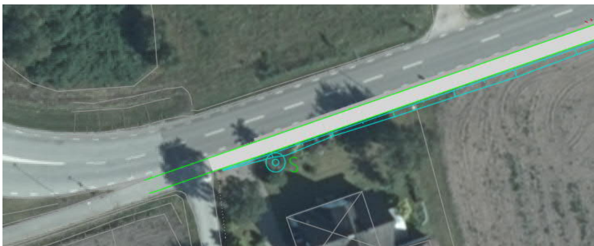
Figur 39. Illustration över vägområde med inskränkt vägrätt
