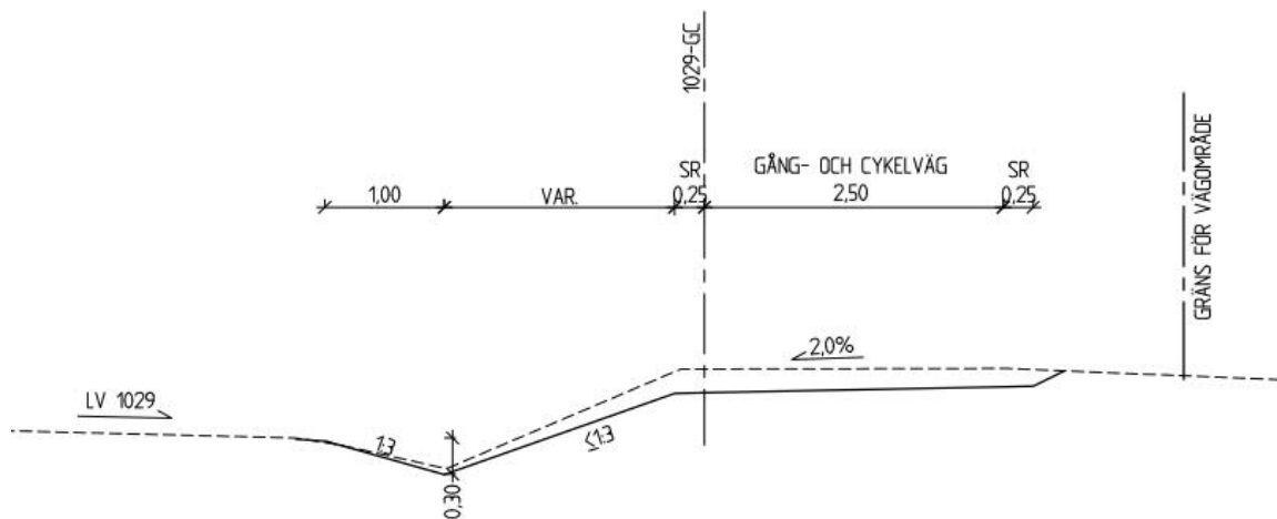
Figur 33. Typsektion, separering med skiljeremsa och svackdike
