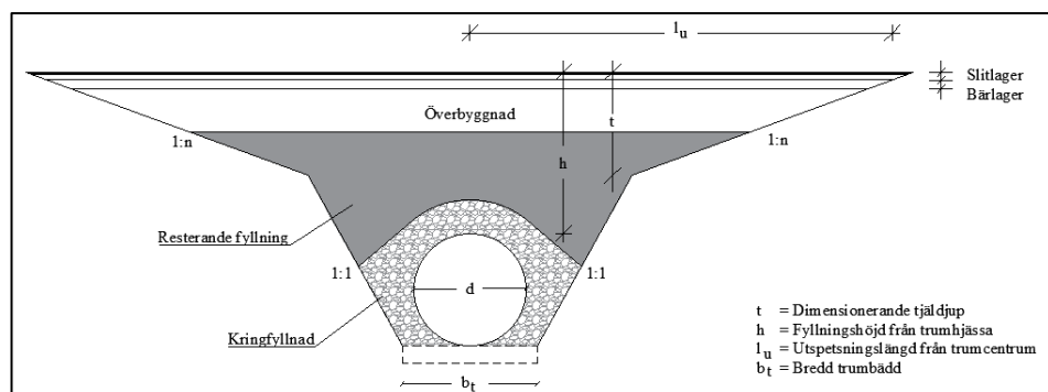
Figur 83.173b Principskiss trumma förlagd under dimensionerande tjäldjup
