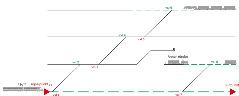
Figur 1. Bilden visar ett exempel på hur kravet på motväxlarna kan uppfyllas. För att tåg 11 ska få passera signalpunkt yy med ett stoppassagemedgivande ska dels växel 7, dels minst en av växlarna 1, 3 och 5 ligga i ett läge som skyddar andra tåg eller spärrfärder (annan rörelse). De skyddande växlarna ska också vara låsta.
