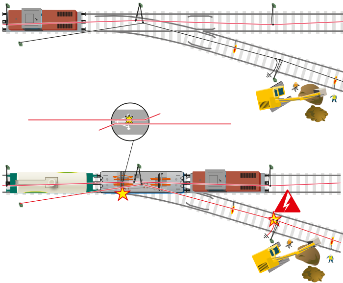
Figur 1. Vid arbete på eller i närheten av kontaktledningen ska denna vara fränkopplad, spänningsprovad och arbetsjordad för att inte orsaka livsfara. Men en spänningslös kontaktleddning kan plötsligt göras spänningsatt av ett elfordon genom överbrygning.
