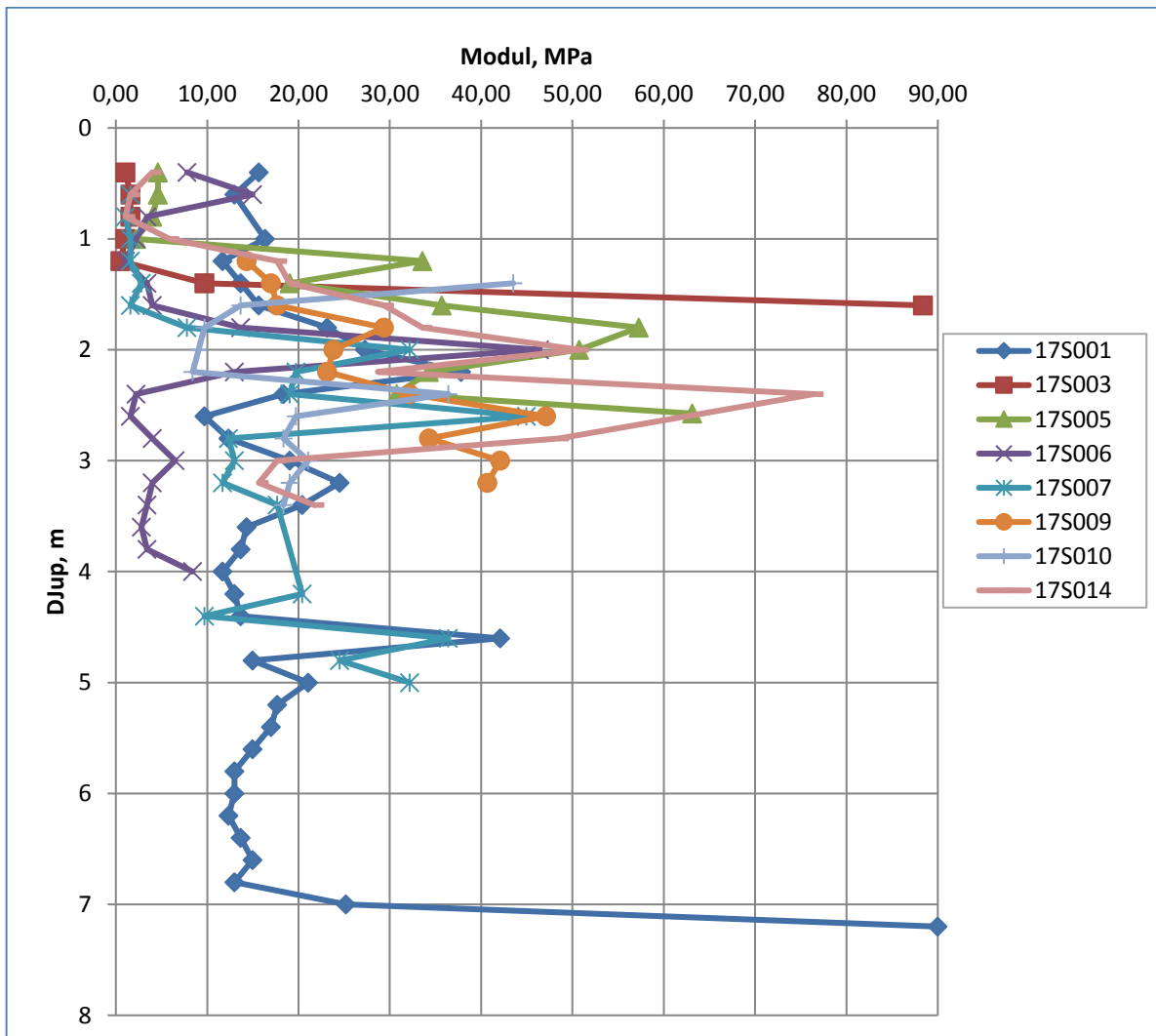
Figur 8.1.2 Härledda värden elasticitetsmodul
