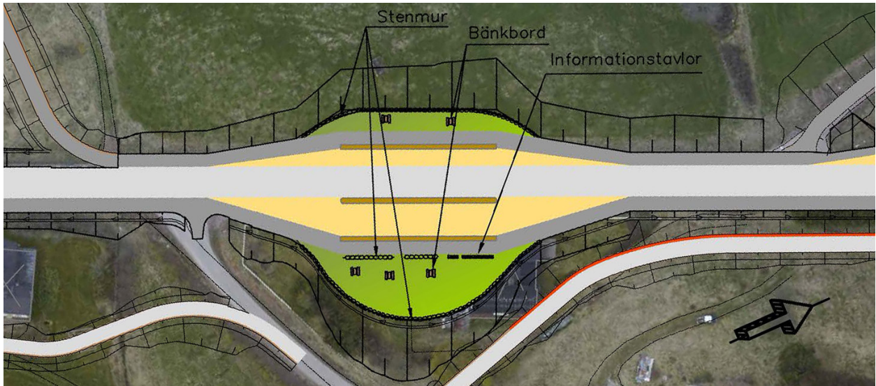
Förslag på utformning av utsiktsplatsen.
