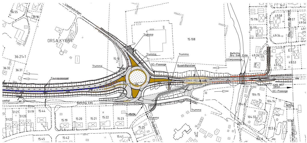
Föreslagna åtgärder på delsträcka 3, närmst Orsa.
