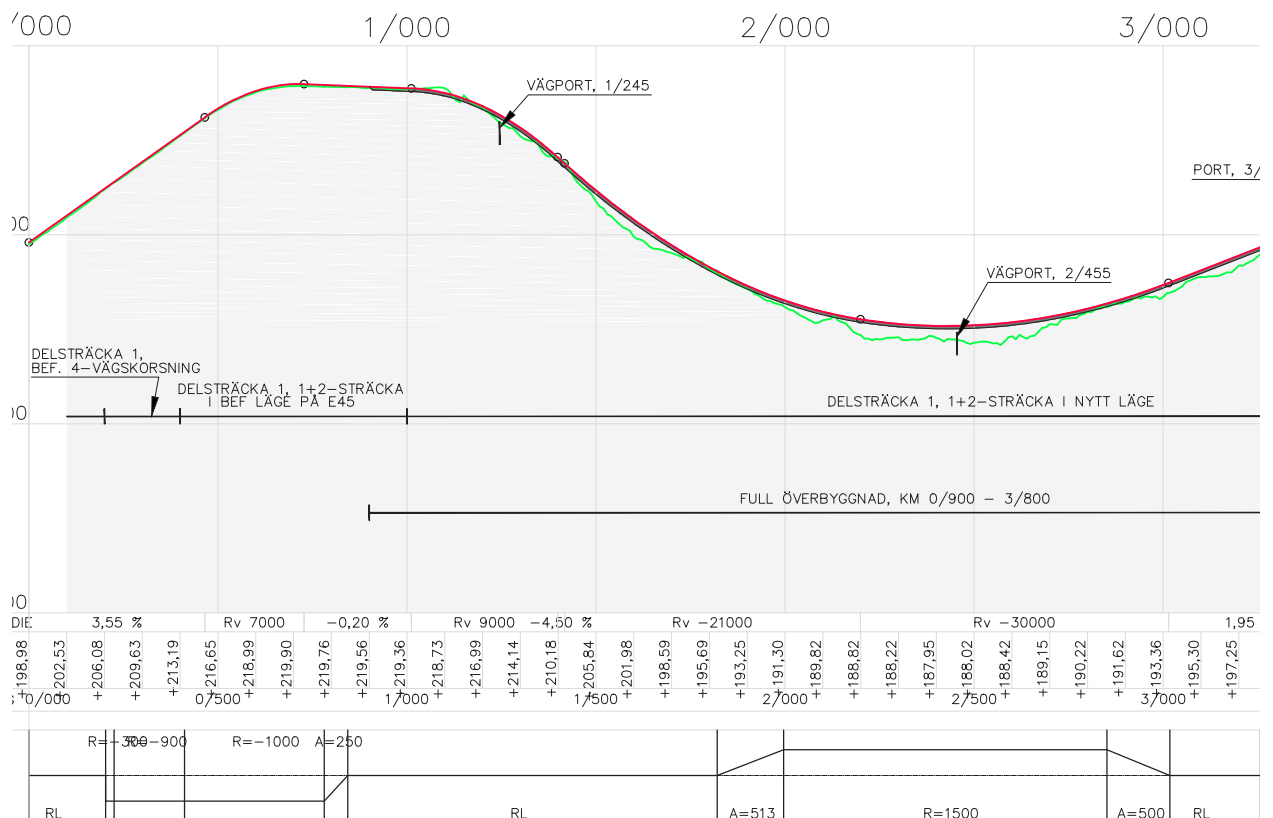
Vägens plan och profil i södra delen.
