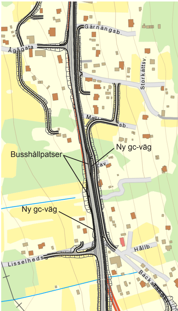
Föreslagen väglinje och åtgärder på delsträcka 2 genom Holen
