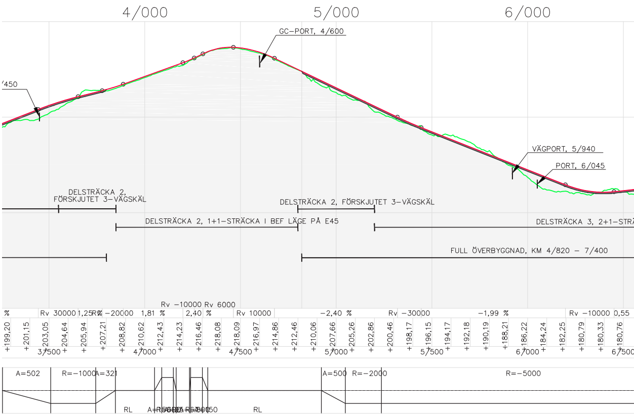
Vägens plan och profil i norra delen.
