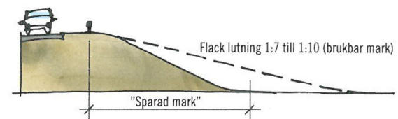
Överskottsmassor kan användas till att göra flacka banksslänter. Det kan bidra till att man slipper använda räcke samt kan göra jordbruksmark brukbar.
