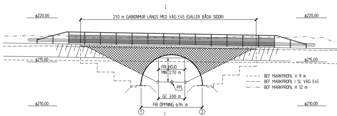
Bro över gc-väg i Holen km 4/610
