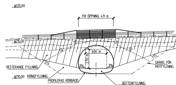
Föreslagen gc-port vid km 1/246
