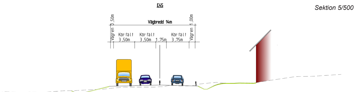
Föreslagna åtgärder på delsträcka 3, närmst Orsa.
