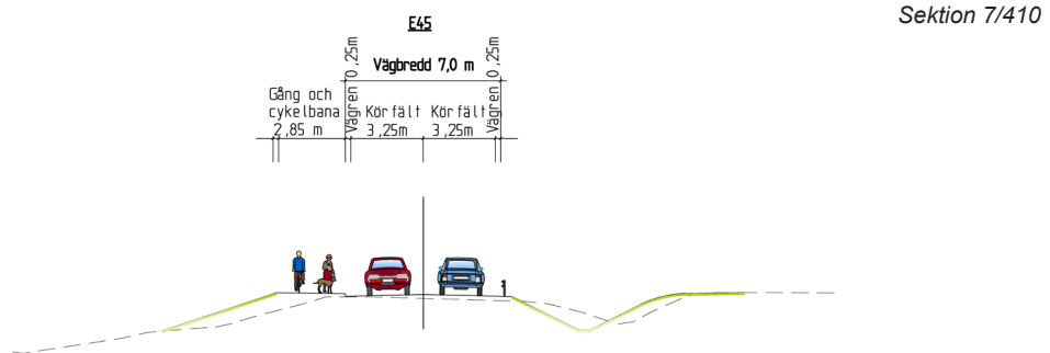
Föreslagna typsektioner, delsträcka 3.
