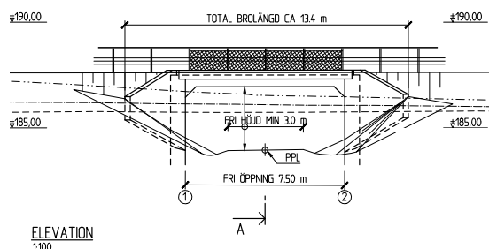
Föreslagen bro och viltpassage vid km 2/458
