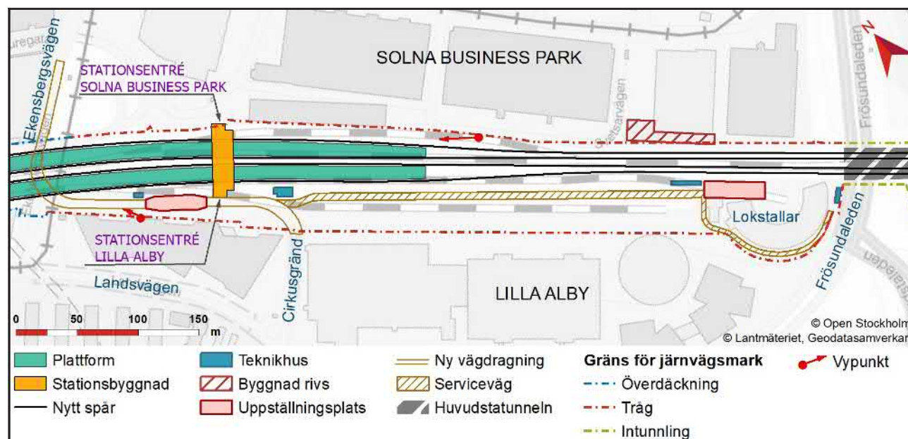
Figur 32. Karta över anläggningsdel Tråget.
