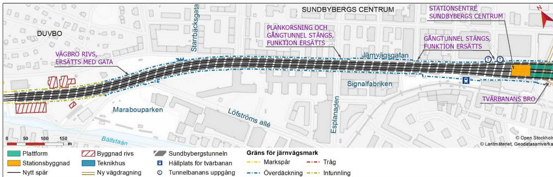
Figur 35. Karta över anläggningsdel Sundbybergstunneln.
