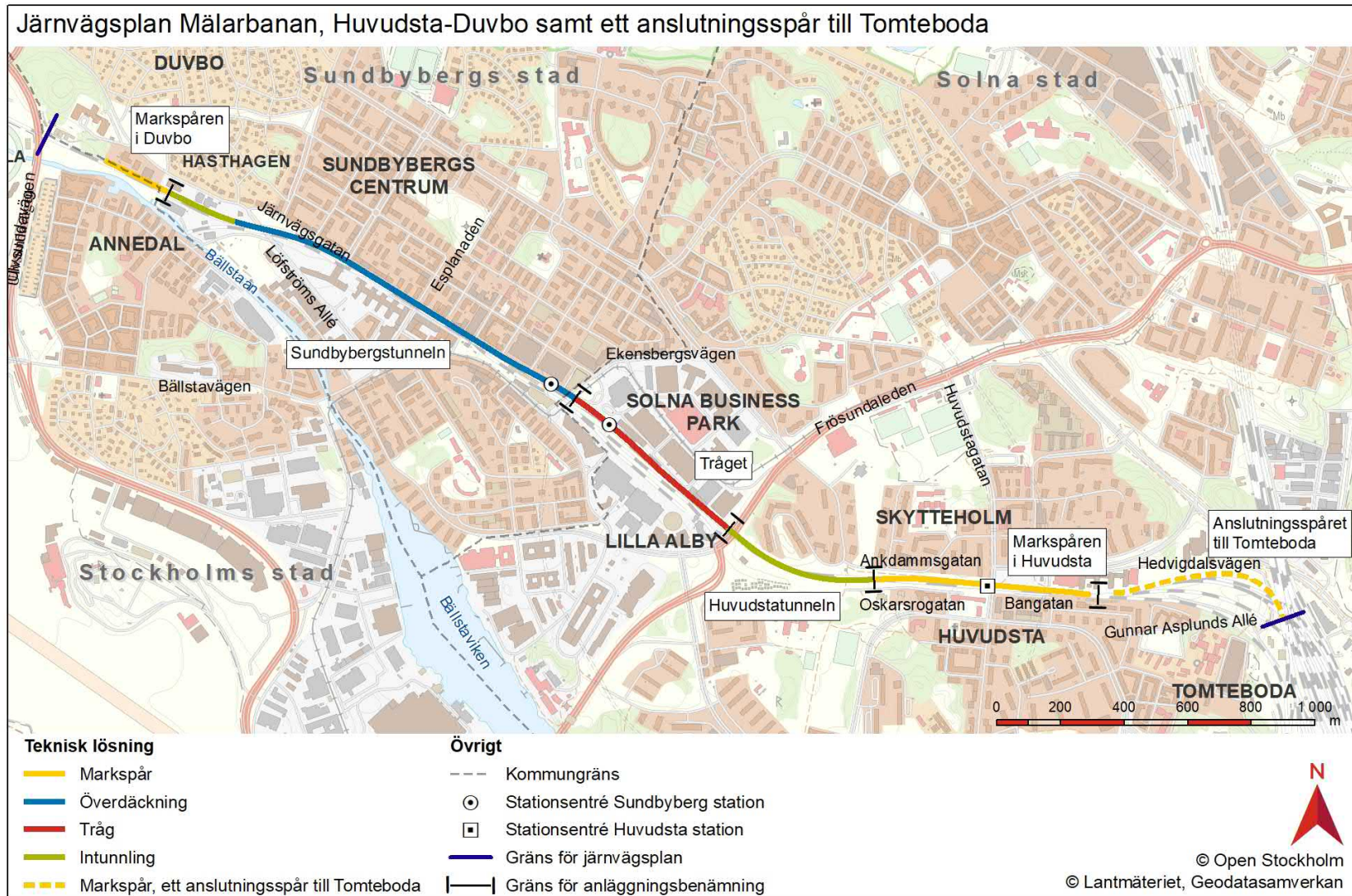
Figur 24. Järnvägsutbyggnaden Mälarbanan delsträcka Huvudsta-Duvbo.
