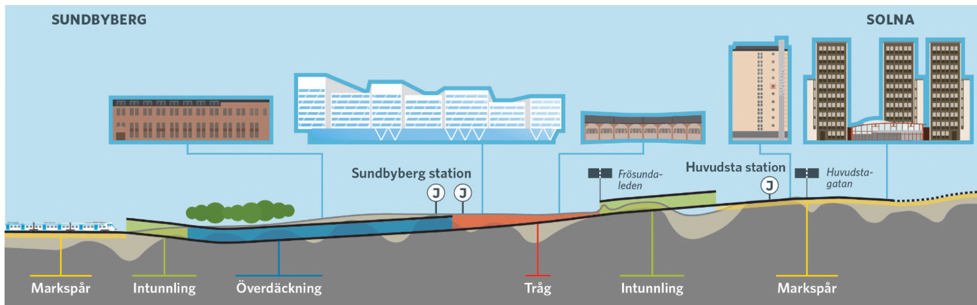
Figur 23. Schematisk längdprofil för Mälärbanan delsträcka Huvudsta-Duvbo samt placering av järnvägen i förhållande till kringliggande marknivå.
