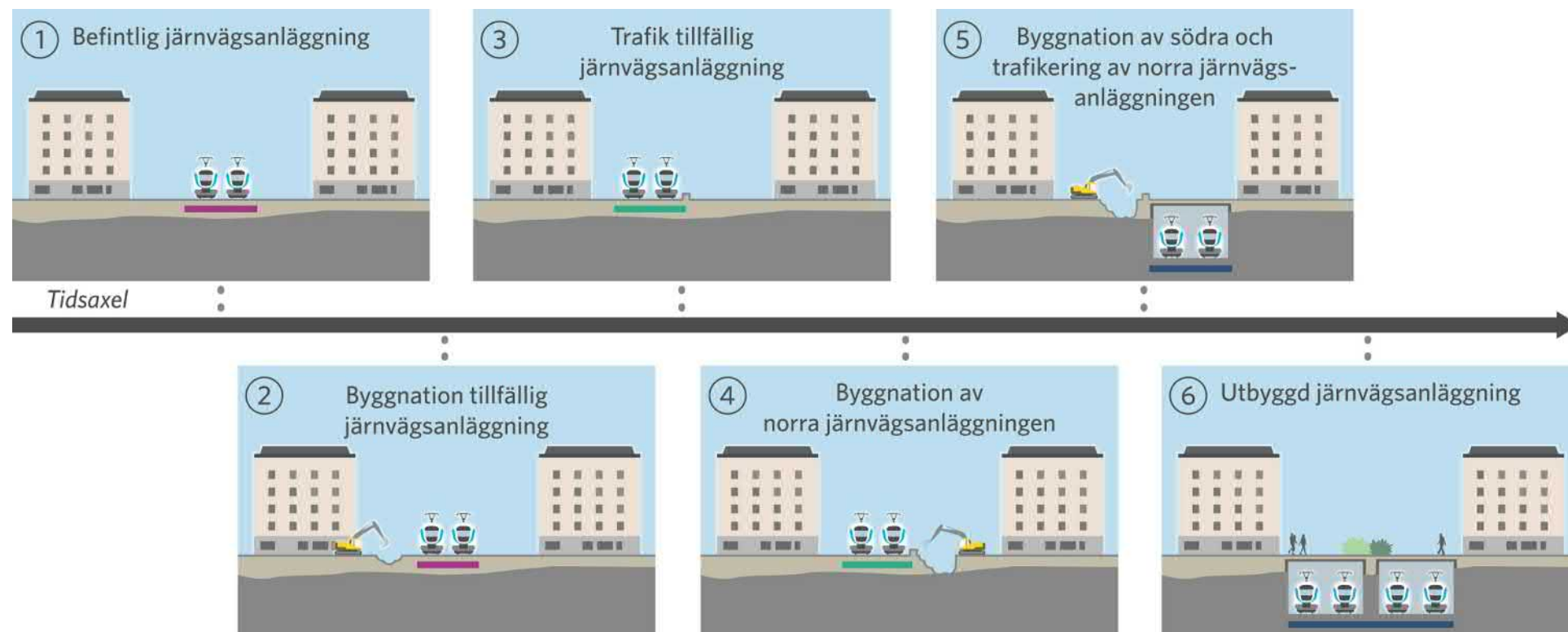
Figur 42. Principbild som visar den stegvisa omläggningen av Mälarbanans trafikering under byggtiden av de två tunnelrören genom Sundbyberg.
