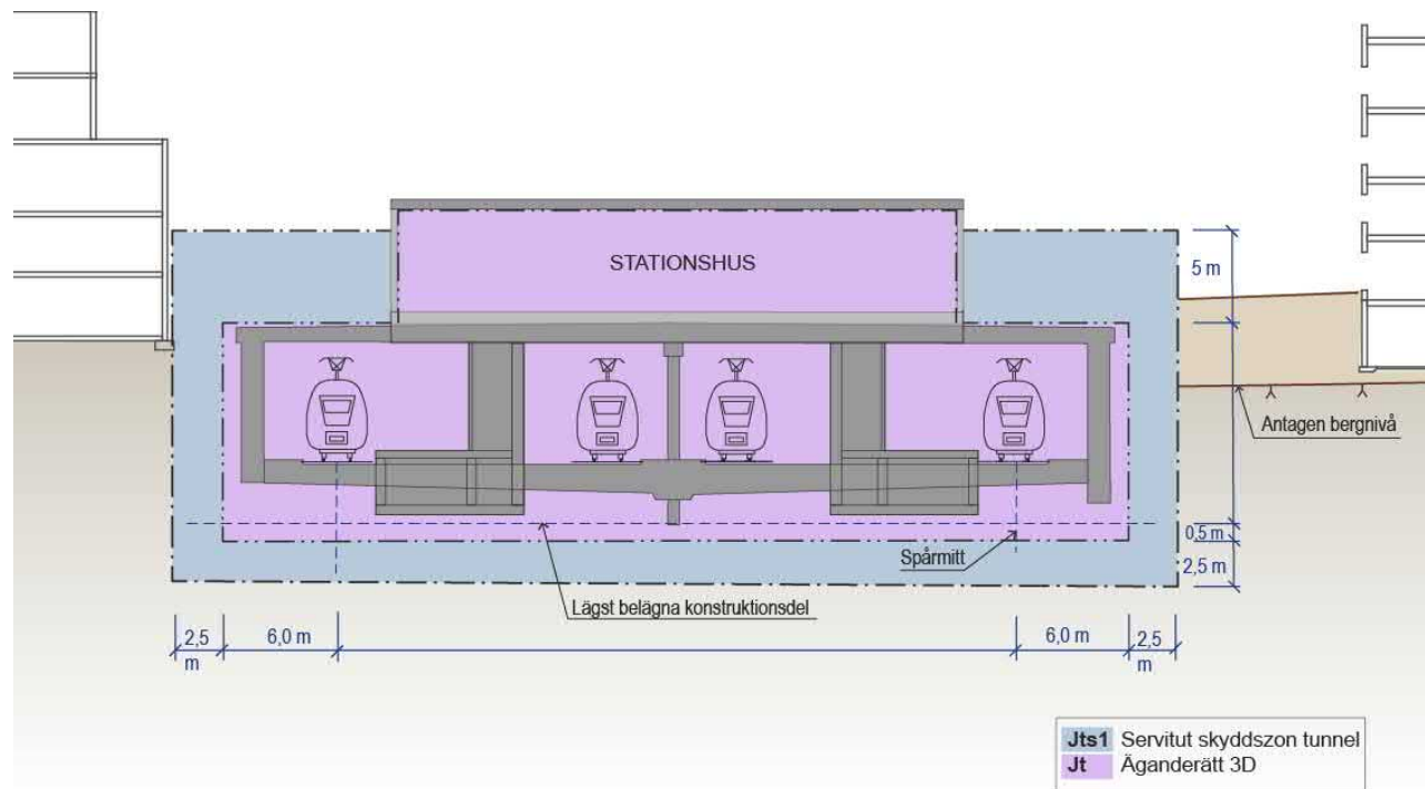
Figur 59. Princip för fastighetsbildning för Sundbyberg stationshus.
