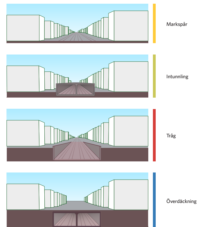
Figur 22. Järnvägsanläggningens fyra tekniska lösningar utmed sträckan. Färgerna kopplar till kartan i Figurena 23 och 24.
