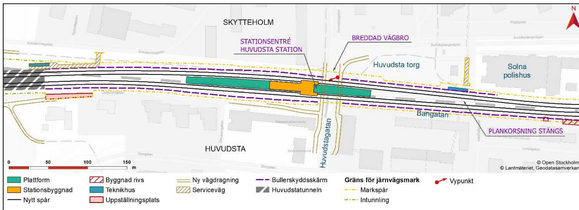
Figur 27. Karta över anläggningsdel Markspåren i Huvudsta.
