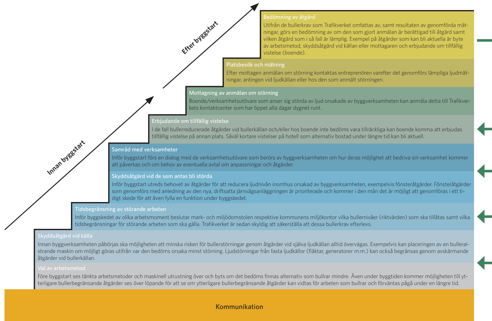
Figur 54. Trafikverket, Projekt Mälarbanans modell för hantering av bullerstörningar under byggskedet.
