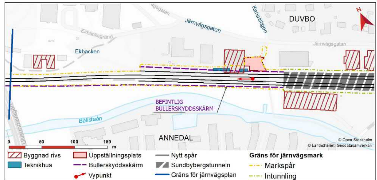
Figur 38. Karta över anläggningsdel Markspåren i Duvbo.
