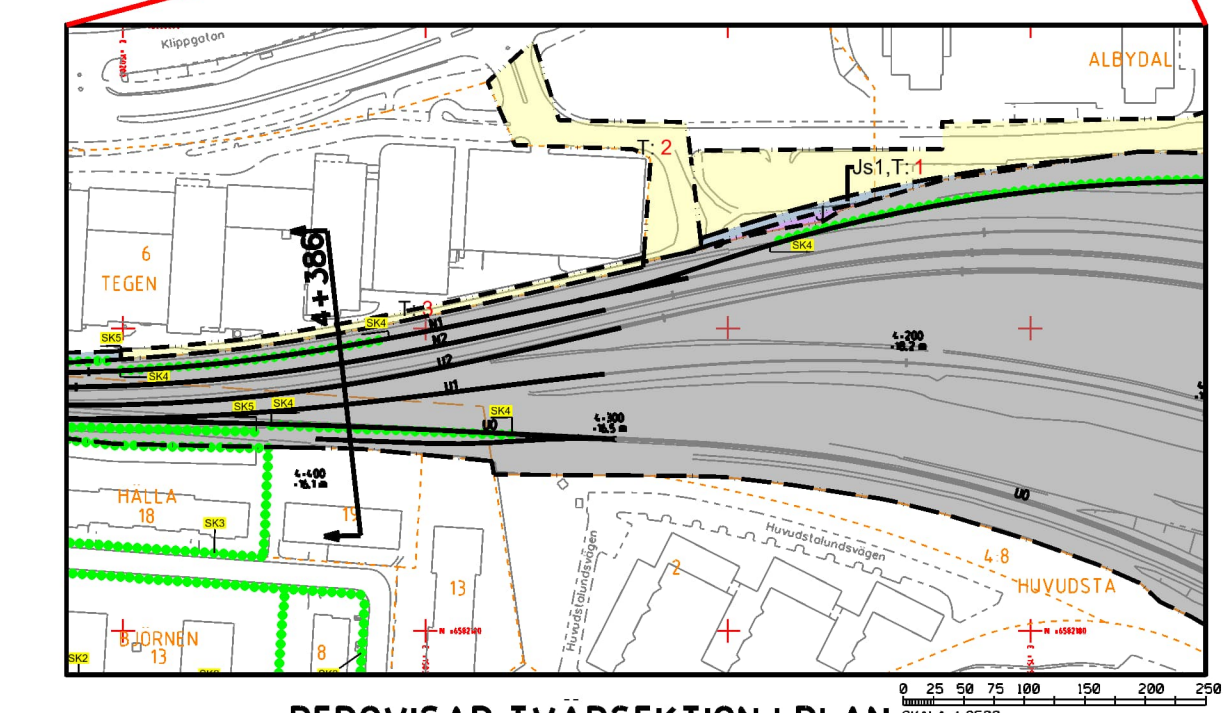
REDOVISAD TVÄRSEKTION I PLAN
