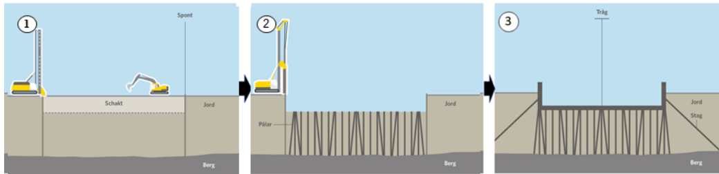
Figur 15. Sekvenser utförande Tråget
