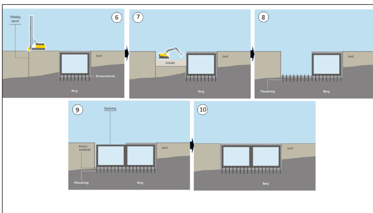
Figur 17. Sekvens som visar byggande av södra tunnelröret Sundbybergstunneln.
