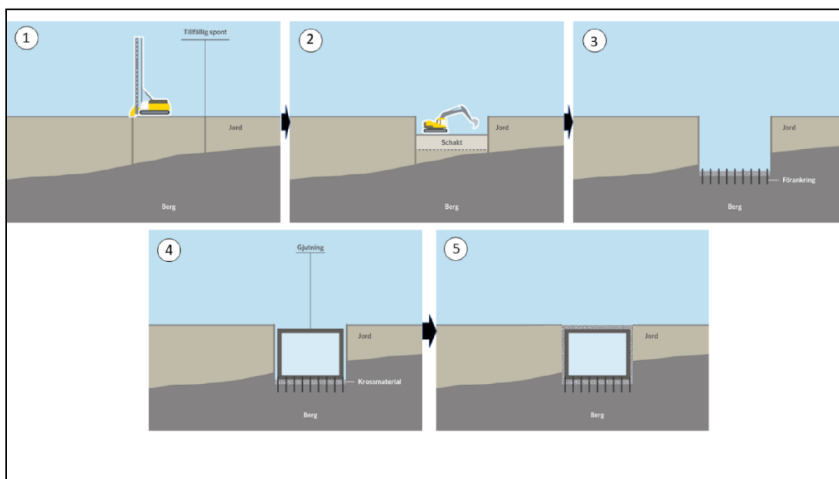
Figur 16. Sekvens som visar byggande av norra tunnelröret Sundbybergstunneln.
