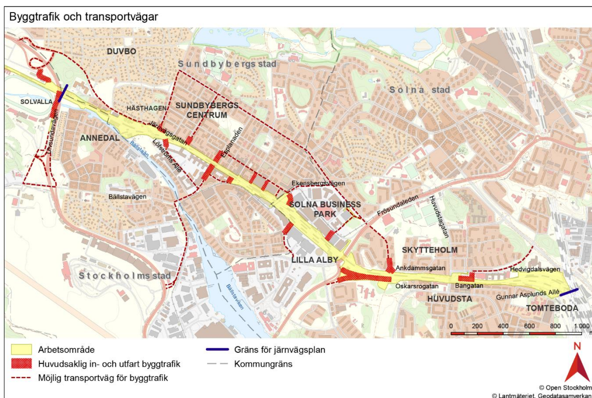
Figur 18. Arbetsområdets in- och utfarter samt möjliga transportvägar för byggtrafik.
