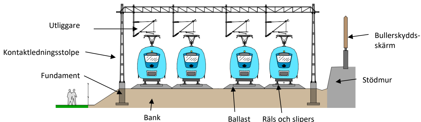
Figur 13. Generell illustration på tvärsektion av järnväg i markplan.
