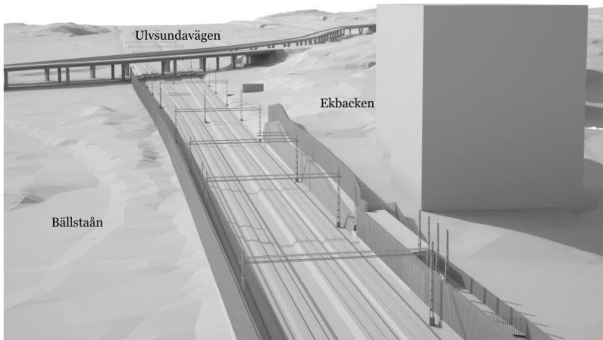
Figur 5. Gestaltungsforlag på markspåren i Duvbo. Bilden är tagen från öster och man ser spåren väster ut.
