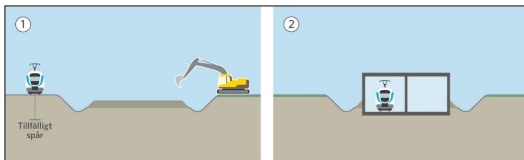
Figur 14. Schematisk skiss Huvudstatunnelns byggskede.
