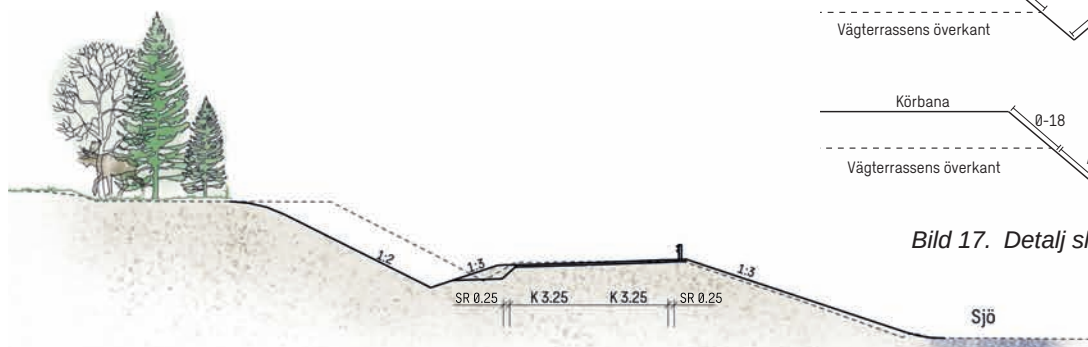
Bild 16. Typsektion väg vid vattendrag
