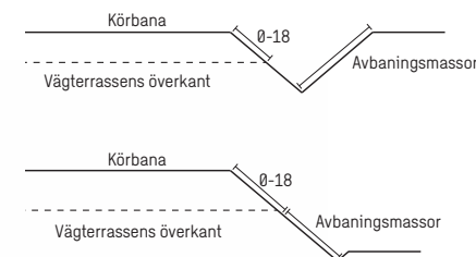
Bild 17. Detalj släntutformning
