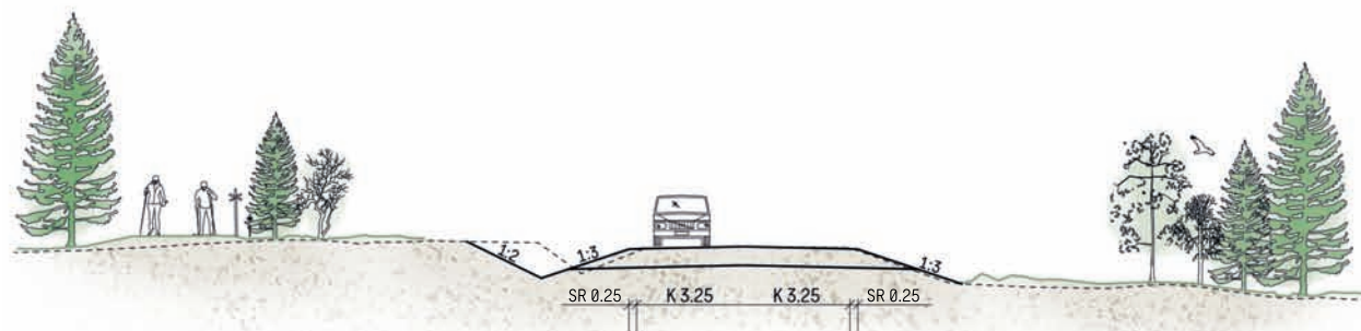
Bild 9. Typsektion väg 1025
