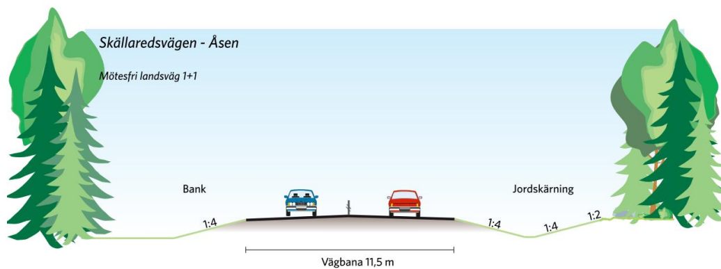
Figur 12 Förenklad typsektionsritning mötesfri landsväg 1+1
