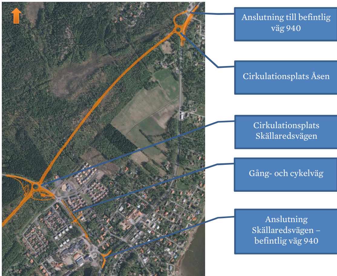
Figur 6 Väg 940, del Skällaredsvägen-Åsen (2 04) anslutning mot befintlig väg 940
