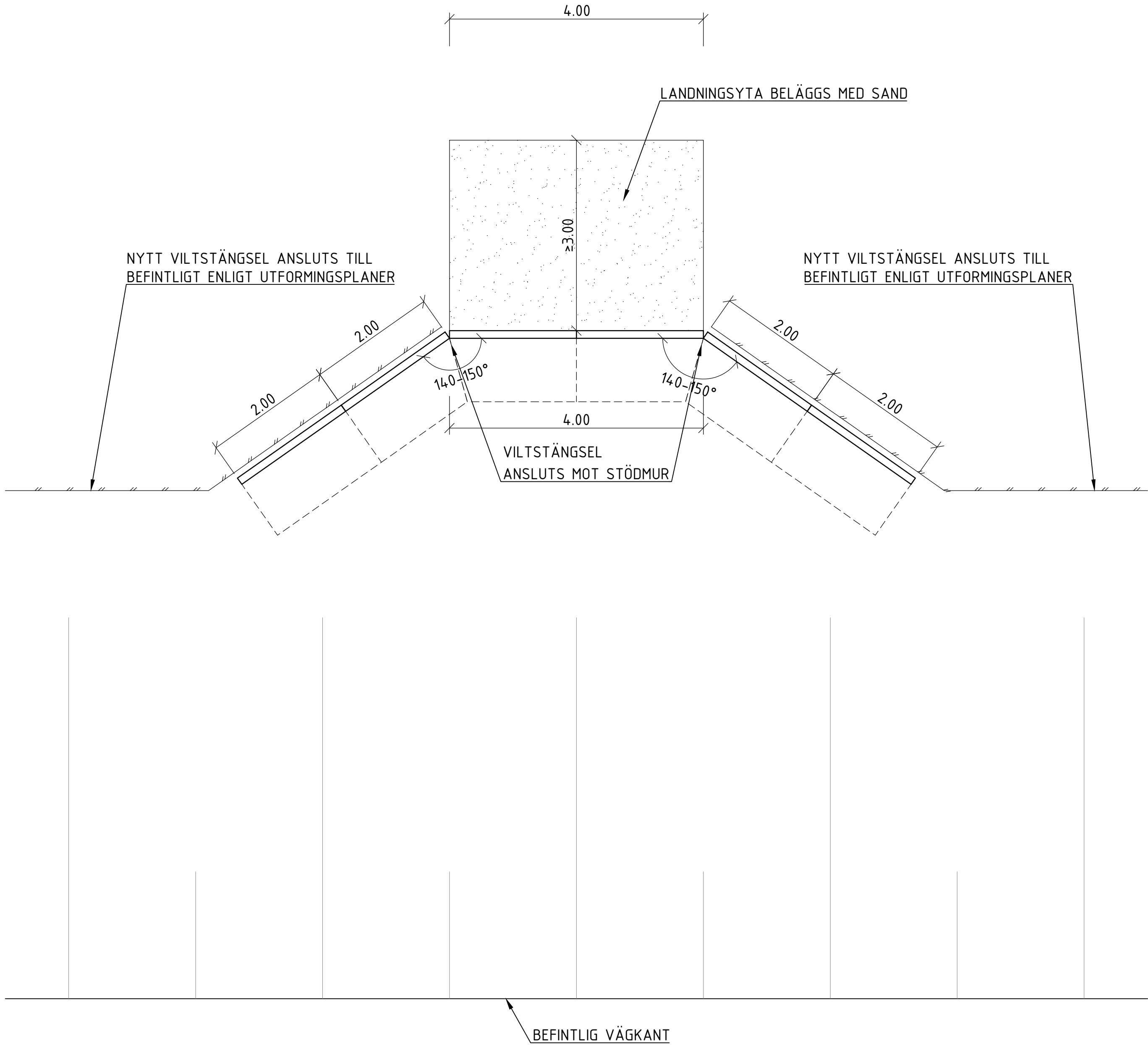
VILTUTHOPP PLAN - ALT 2 SKALA 1:50
