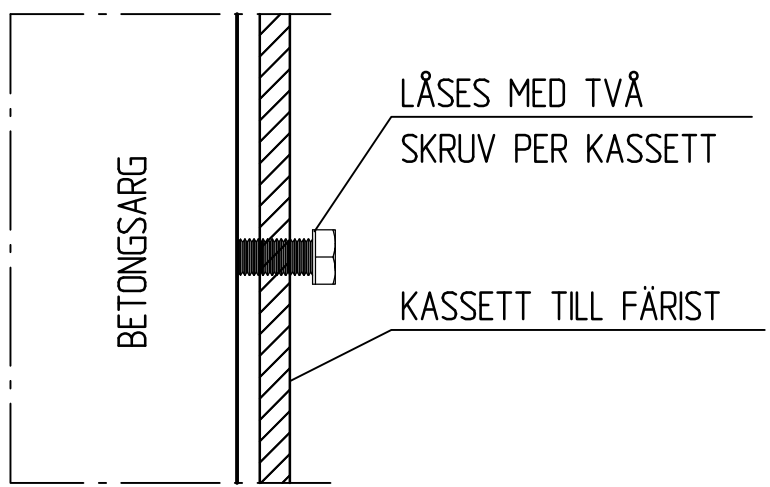
DETALJ, LÄSNING AV KASSETT, PLAN 15
