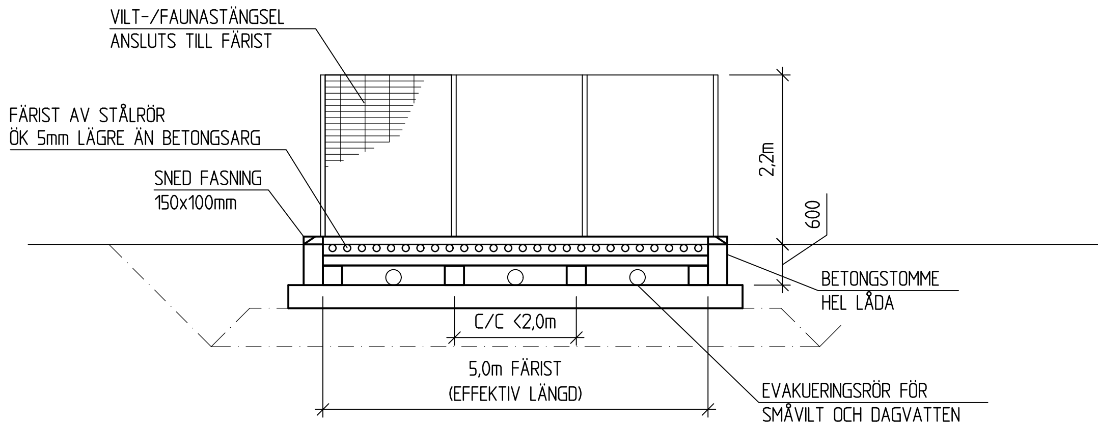
SEKTION A-A 150
