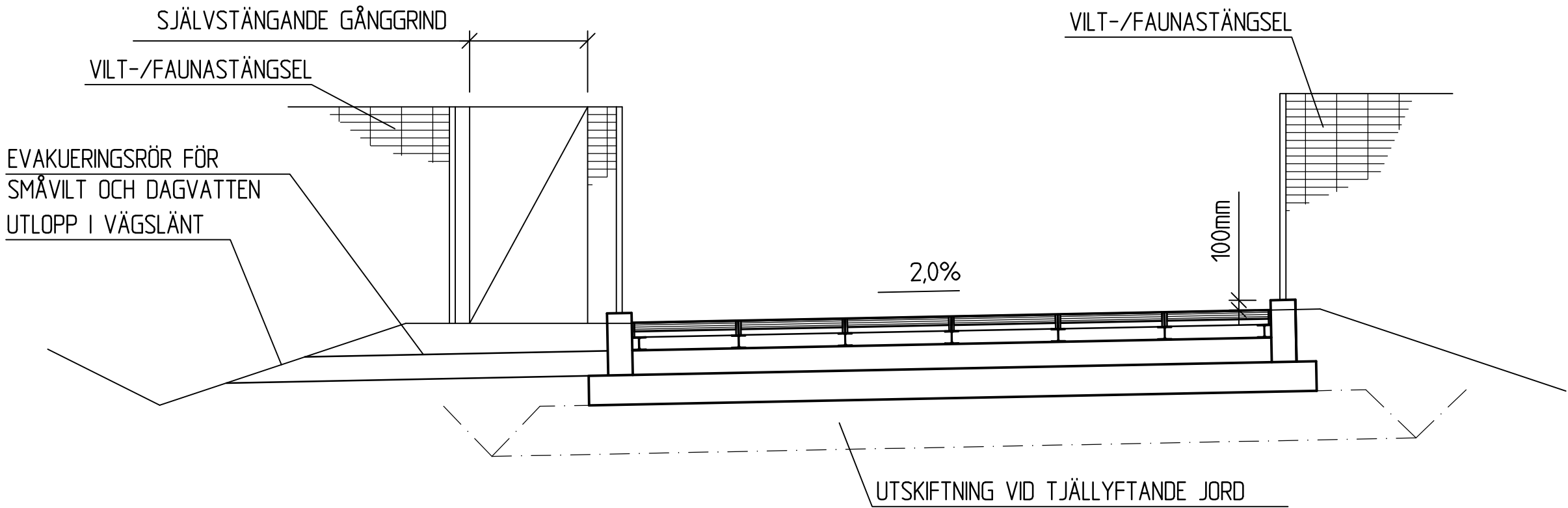
SEKTION B-B 150
