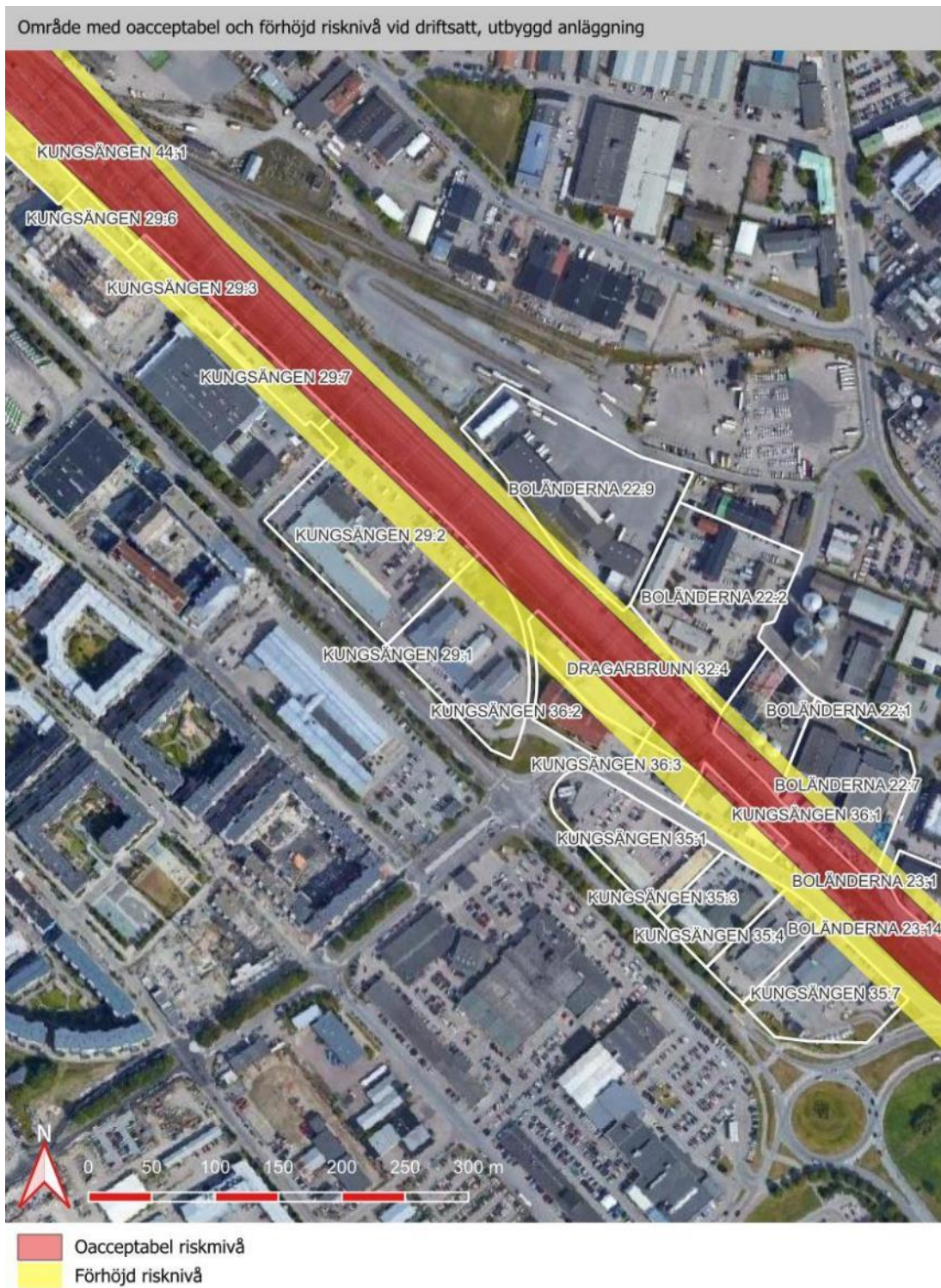
Figur 30. Område i Kungsängen och Boländerna med oacceptabel och förhöjd risknivå vid driftsatt, utbyggd anläggning.
