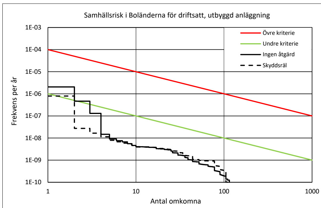
Figur 14. Samhällsrisk i Boländerna för driftsatt, utbyggd anläggning med eller utan föreslagna åtgärder.
