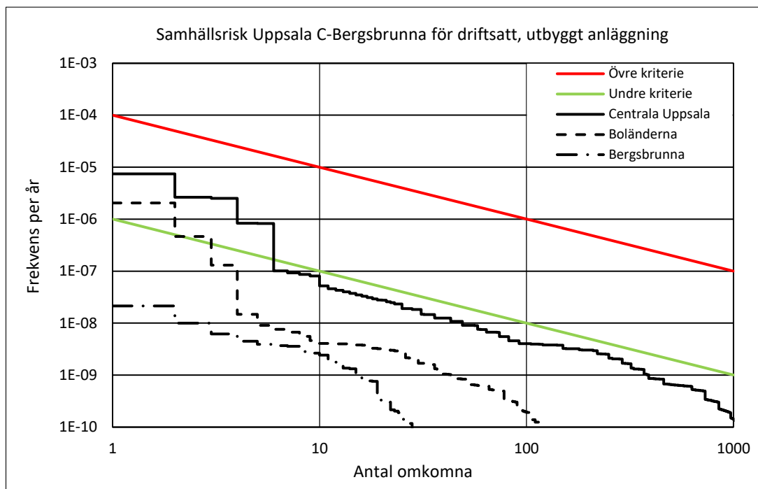
Figur 7. Samhällsrisk längs med 1 kilometer av järnvägsanläggningen i centrala Uppsala, Boländerna och Bergsbrunna, utan hänsyn till skyddsåtgärder.
