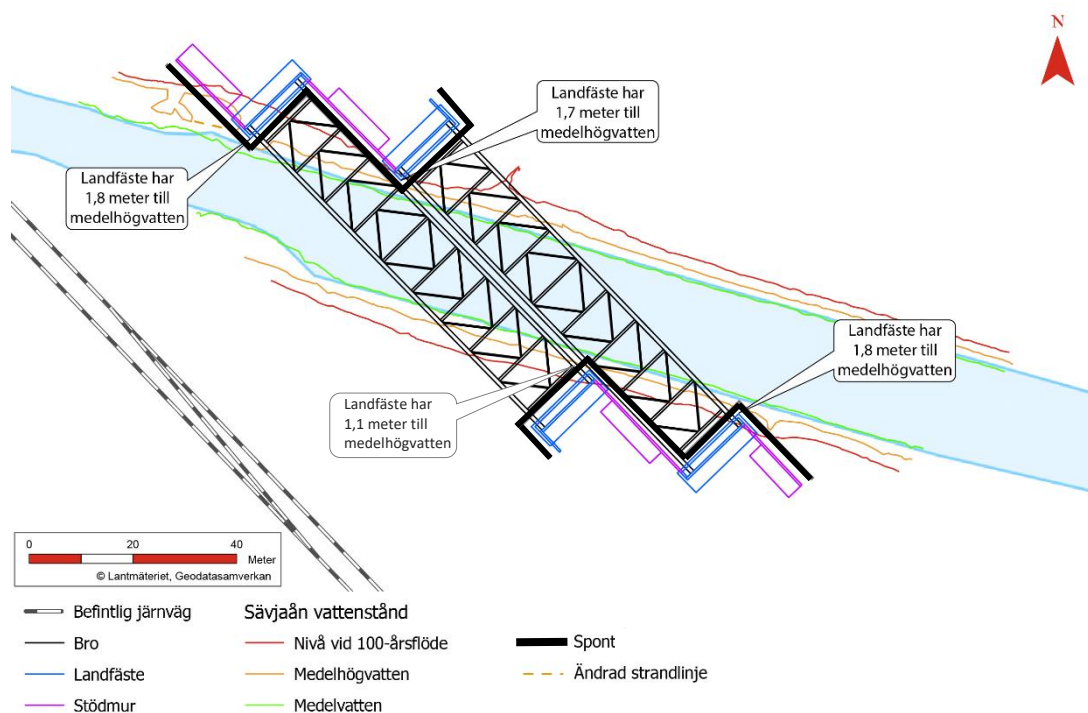
Figur 5. Placering och utformning av planerade broar. Mått i figuren avser avstånd (i plan) mellan brostöd och strandlinjen vid medelhögvatten från de hörn av landfästena som är närmast vattnet. Befintliga spår som rivs syns i figurens vänstra del. I figuren visas också med orange streckad linje i bildens övre vänstra del hur strand som har eroderat bort tidigare planeras att återställas vid det nordvästra brostödet, för att möjliggöra passage för landlevande djur även vid medelhögvatten.
