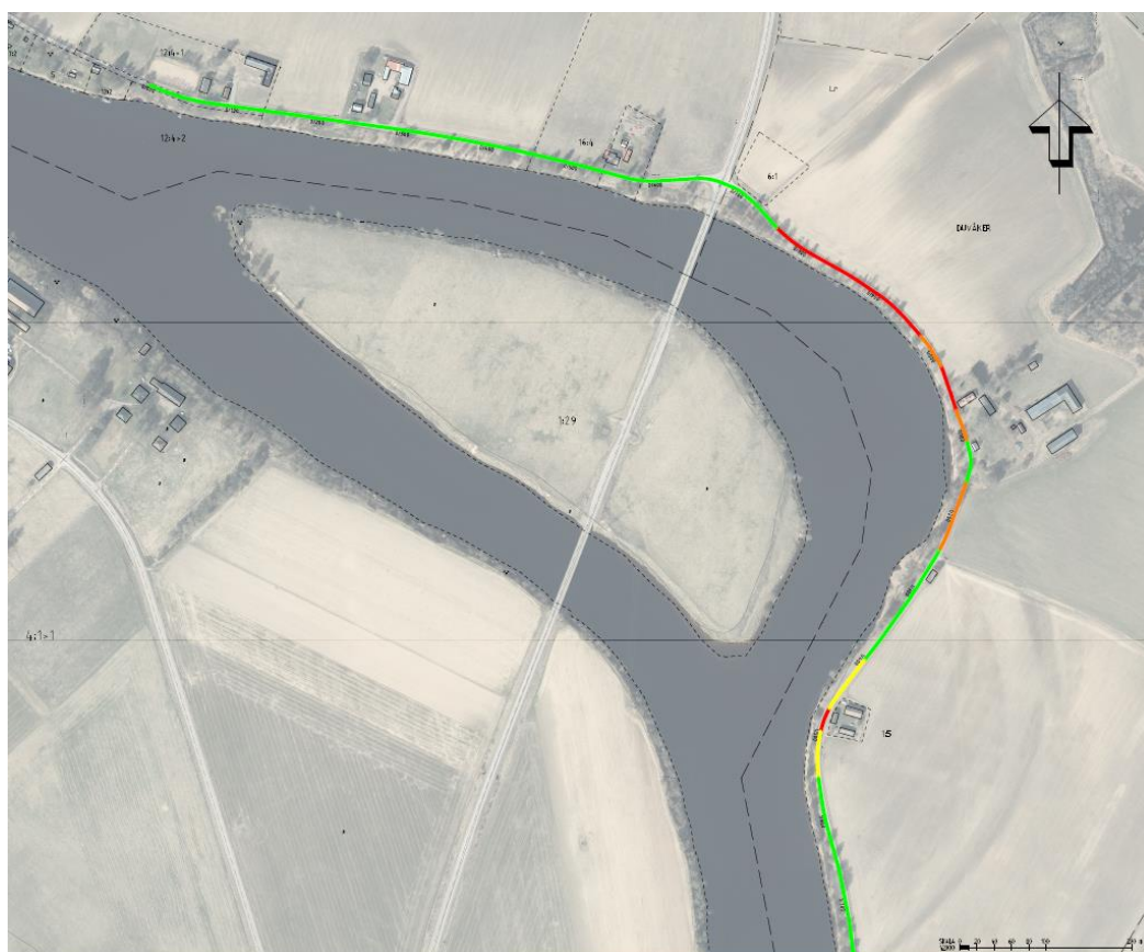
Figur 12. Linjen visar befintlig stabilitet. Färgförklaring: Grön = bra, Gul = OK, Orange = Dålig och Röd = Väldigt dålig. De norra sträckande linjerna visar var vägens läge skulle få en ok eller bra stabilitet.
