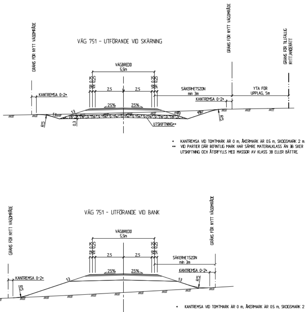
Figur 24. Principutformning av väg.
