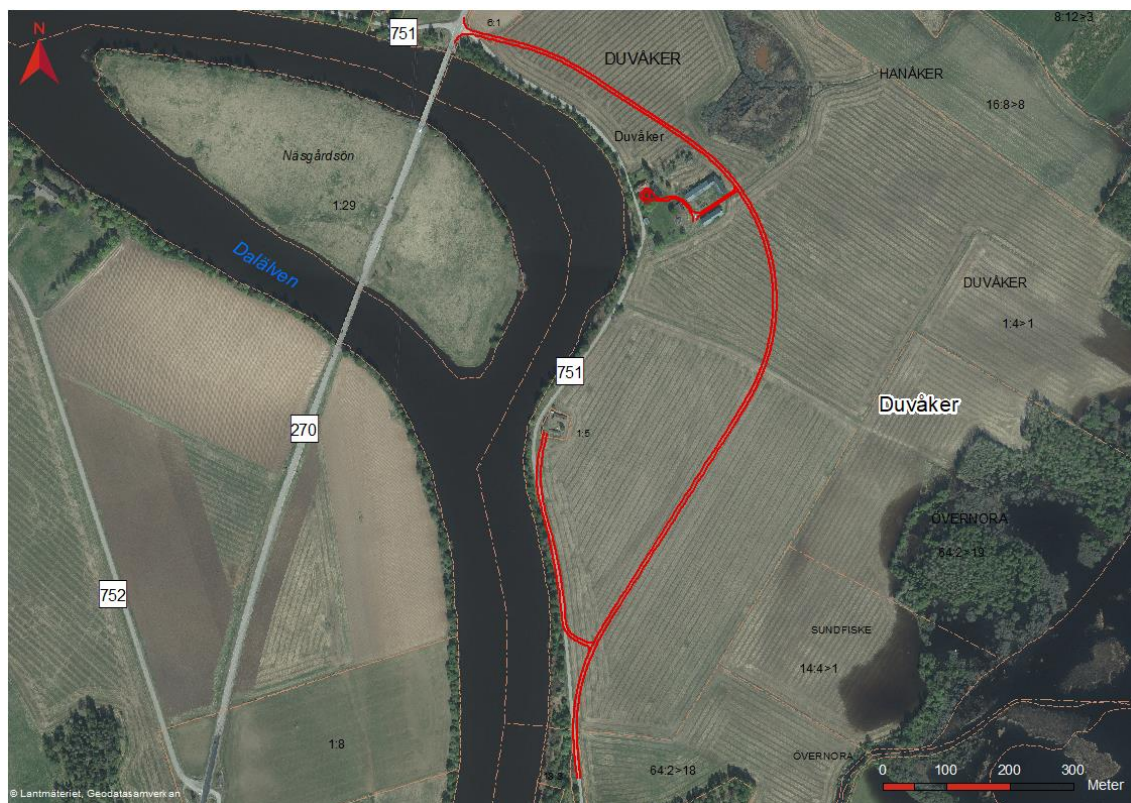
Figur 22. Föreslagen ny lokalisering av väg 751 utmed Duvåker med anslutningsvägar till bostäder.
