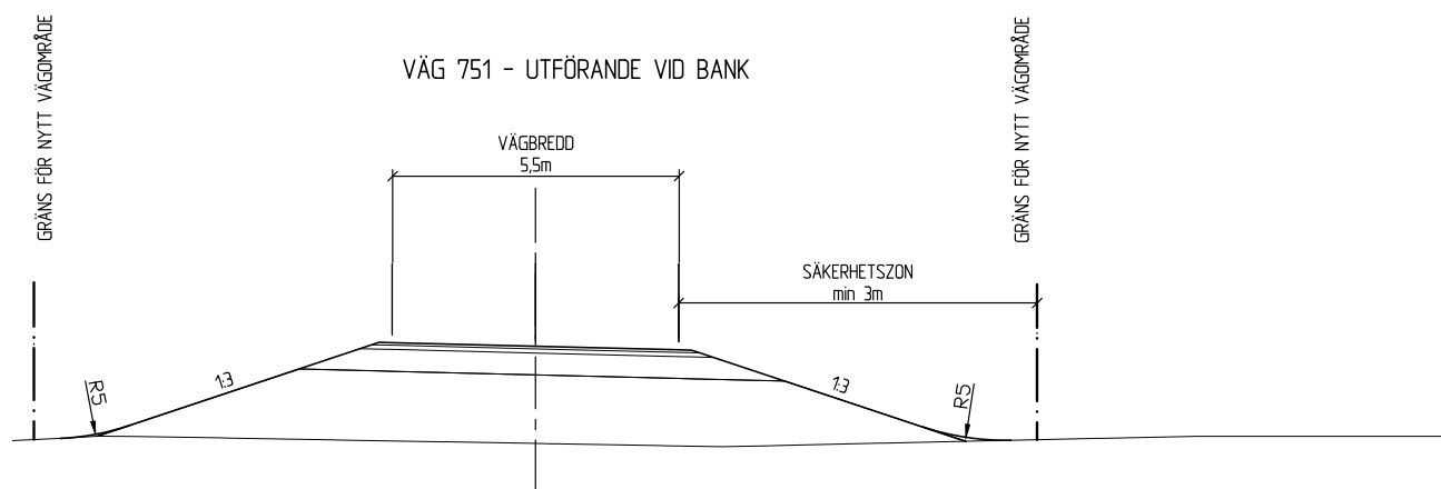
Figur 13. Typsektion Jakobs
