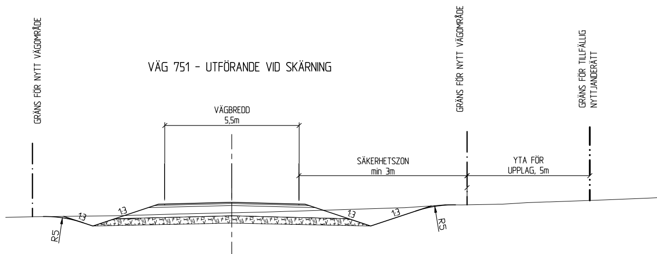
Figur 13. Typsektion Jakobs
