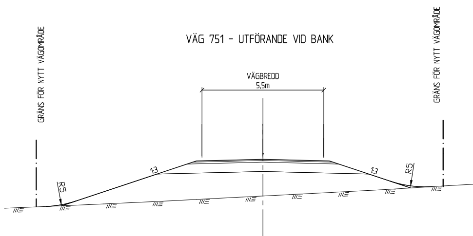
Figur 12. Typsektion Duvåker
