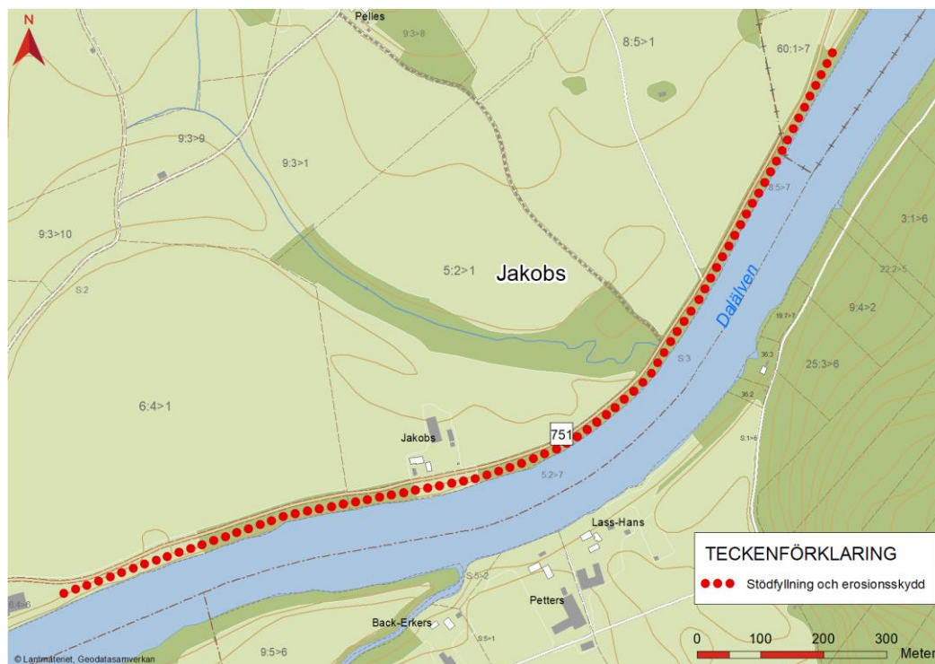
Figur 6 Aktuell sträcka i Jakobs för stödfyllning och erosionsskydd.
