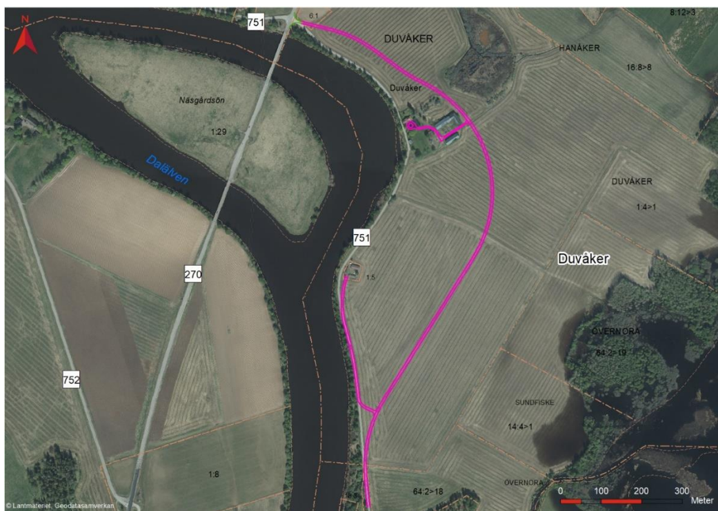
Figur 21 Förordat riskreducerande alternativ i Duvåker, illustrerad med föreslagna förändringar utifrån alternativ Turkos.
