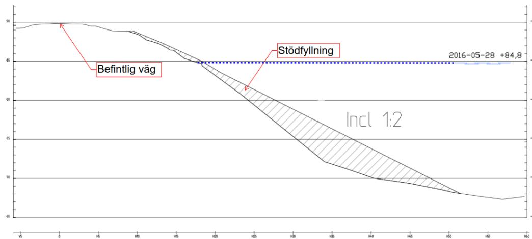
Figur 5 Princip för stödfyllning med erosionsskydd för Jakobs, Myckelby och Duvåker.
