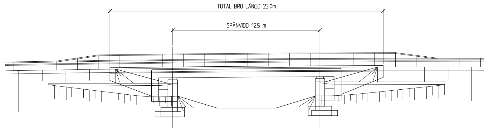
ELEVATION A-A 1:100
