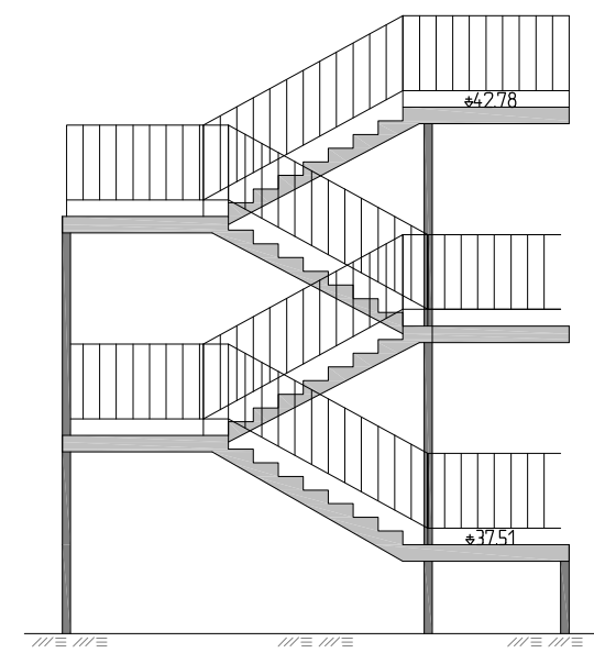
SEKTION TRAPPA 1:50
