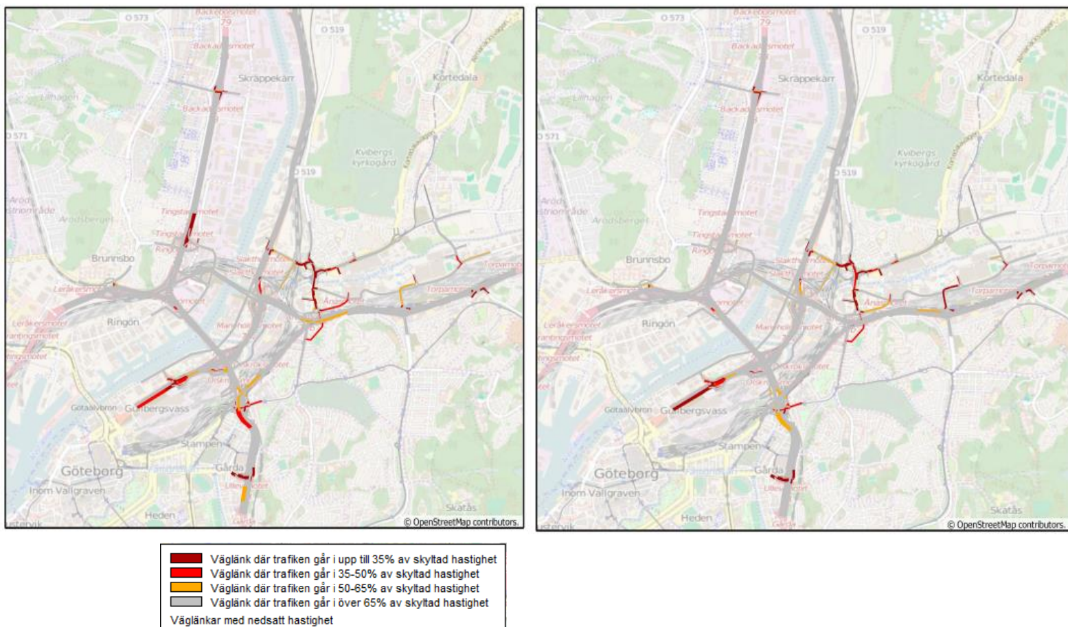
Figur 10: Väglänkar med nedsatt hastighet, när Marieholmstunneln öppnar (vänster bild) respektive om Marieholmstunneln avgiftsbeläggs (höger bild). Dynameq-beräknade resultat.
