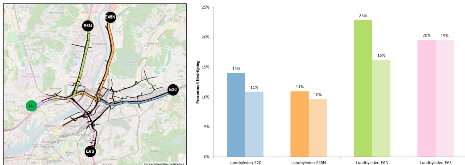
Figur 12: Restidsfördröjningar och varians, under maxtimme, för bilister som startar från Lundbyleden (grön markering). Vänster stapel= Marieholmstunneln utan trängselskatt, höger stapel=Marieholmstunneln med trängselskatt
