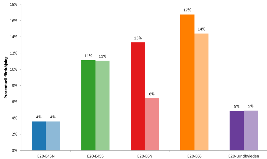
Figur 11: Restidsfördröjningar under maxtimme, för bilister som startar från E20 (grön markering). Vänster stapel= Marieholmtunneln utan trängselskatt, höger stapel=Marieholmtunneln med trängselskatt
