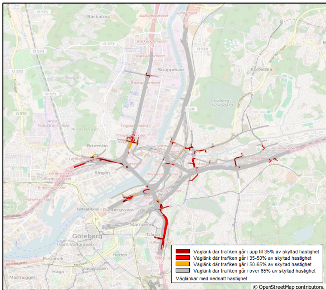
Figur 9: Väglänkar med nedsatt hastighet under eftermiddagens maxtimme. Dynameq-beräknade resultat.
