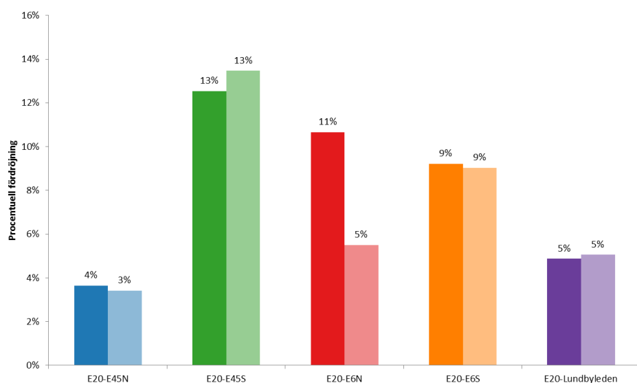
Figur 14: Restidsfördröjningar och varians för bilister som startar från E20 (grön markering). Vänster stapel= Marieholmtunneln utan trängselskatt och stomnät, höger stapel=Marieholmtunneln med trängselskatt och stomnät
