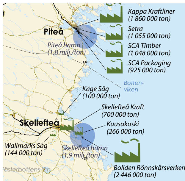
Figur 7.4:1. Större godsgenererande verksamheter mellan Skellefteå och Piteå, ton/år. (Källa: ÅF/Infraplan).
