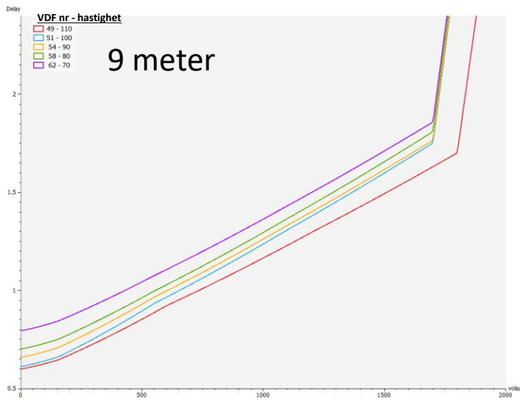
Figur 13. Timme VDF för tvåfältsvägar 9m bredd – olika hastighet
