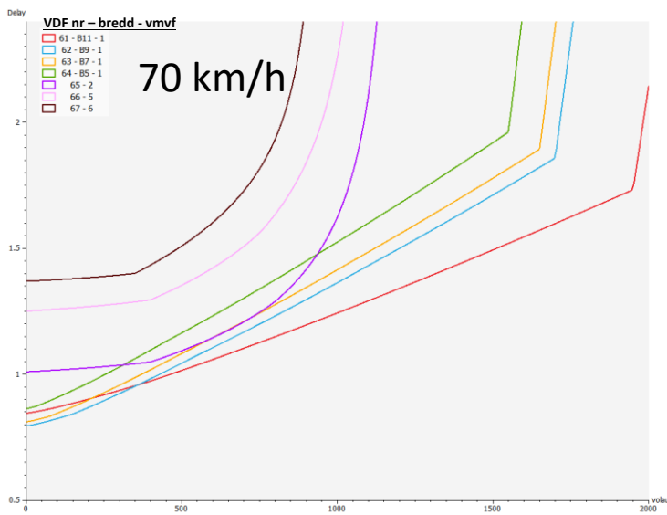
Figur 14. Timme VDF för tvåfältsvägar 70 km/h – olika bredd och vmf
