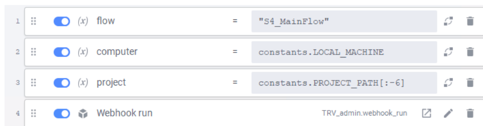
Figur 27. Steg i modulen Webhook
