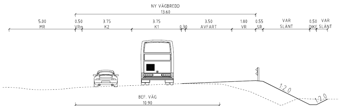
Figur 14 Typsektion
