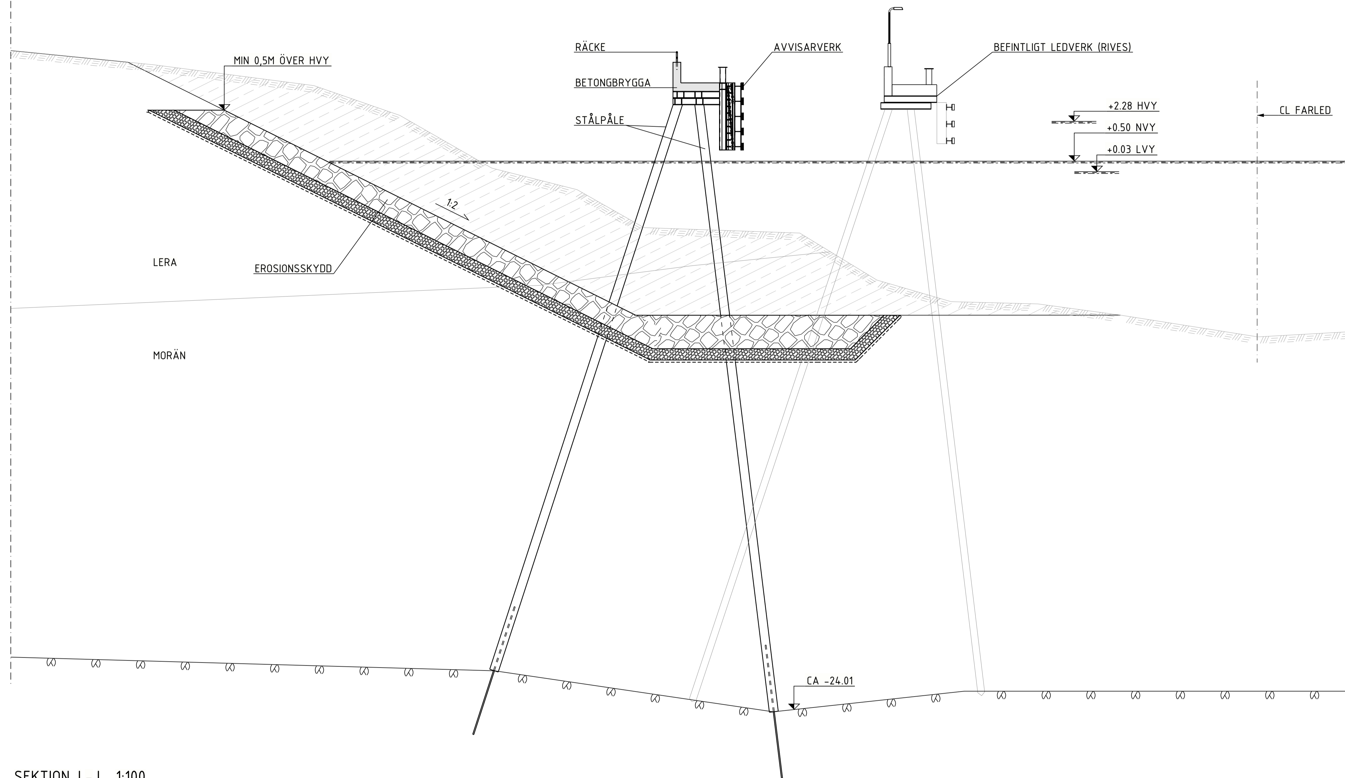
SEKTION I - I 1:100 S.14+TK.T.C00-XDA.R.105
