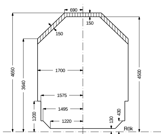
Figur 2.1 Statisk referensprofil A
