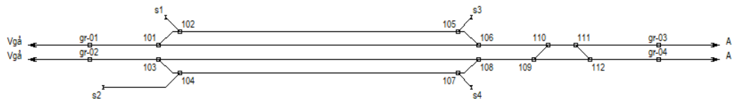
Figur 4 Algutsgården, spårlayout
