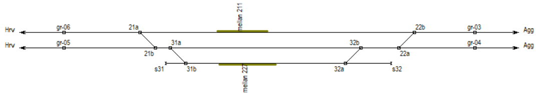
Figur 3 Vårgårda med plattformsplaceringar
