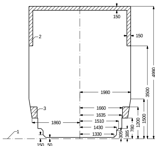
Figur 2.3 Dynamisk referensprofil SEc
