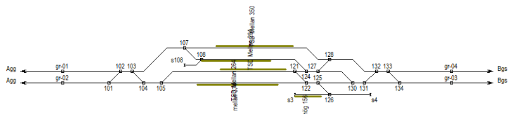
Figur 5 Alingsås
