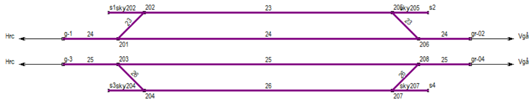
Figur 2 Herrljunga västra
