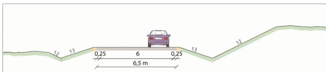
Figur 20. Illustration som visar en sektion för de delar av Slätterödsvägen och Havgårdsvägen som byggs om.
