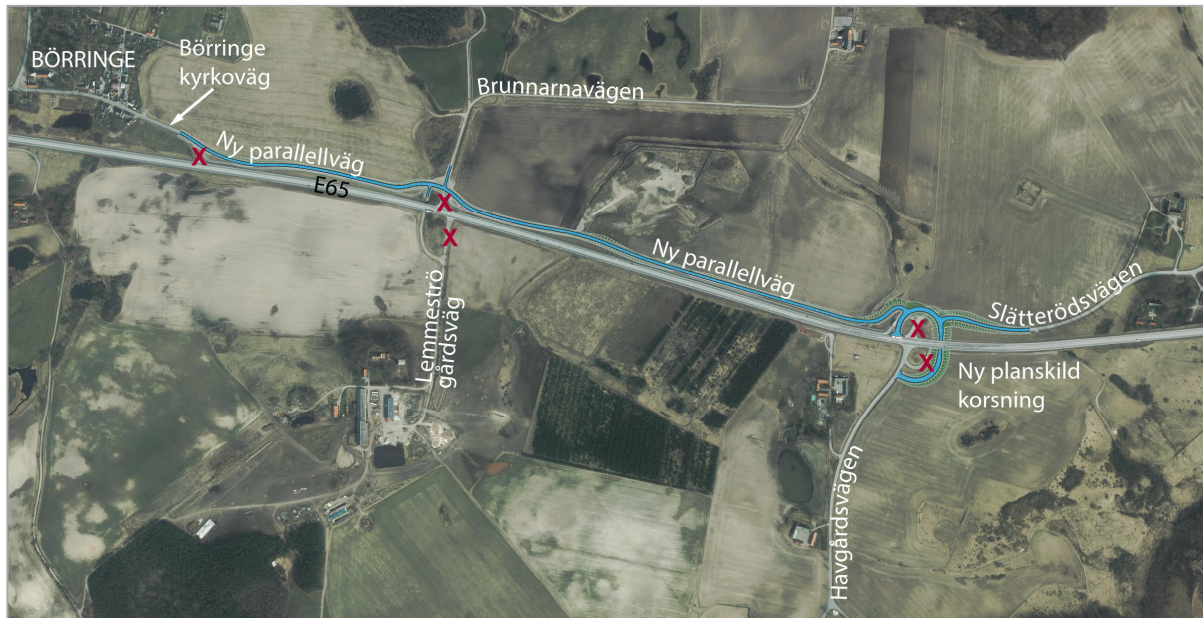
Figur 17. Illustration som visar projektets utbredning, in- och utfarter som stängs samt vändöglor som tas bort då den planskilda korsningen byggs (korsningar och vändöglor är markerade med röda X).
