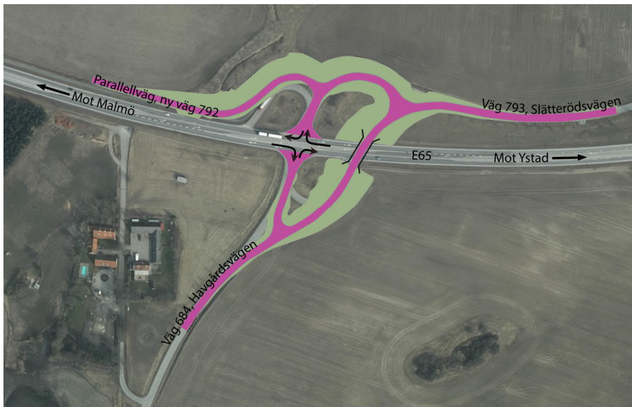
Figur 15. Utformningsexempel med bro över väg E65
