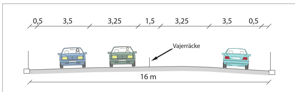
Figur 19. Illustration som visar en sektion med två körfält i vardera riktningen på E65 i den planskilda korsningen. I dag finns ett körfält i vardera riktningen samt vänstersvängskörfält.
