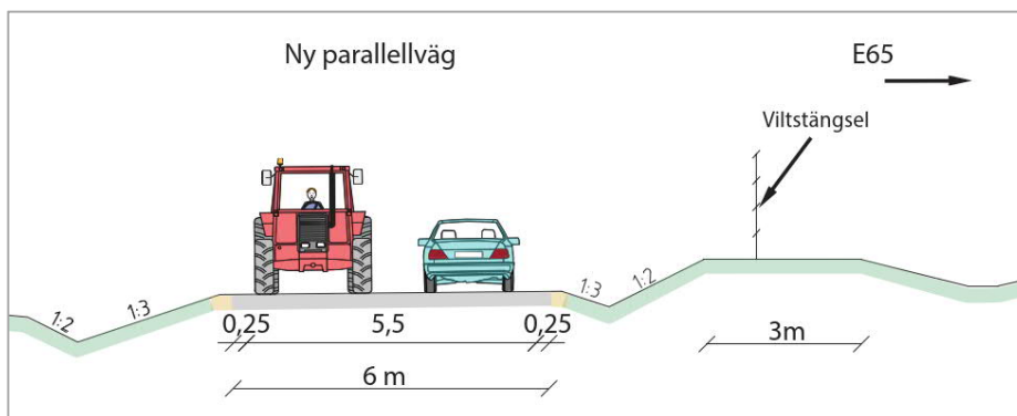
Figur 18. Illustration som visar en sektion av parallellvägen
