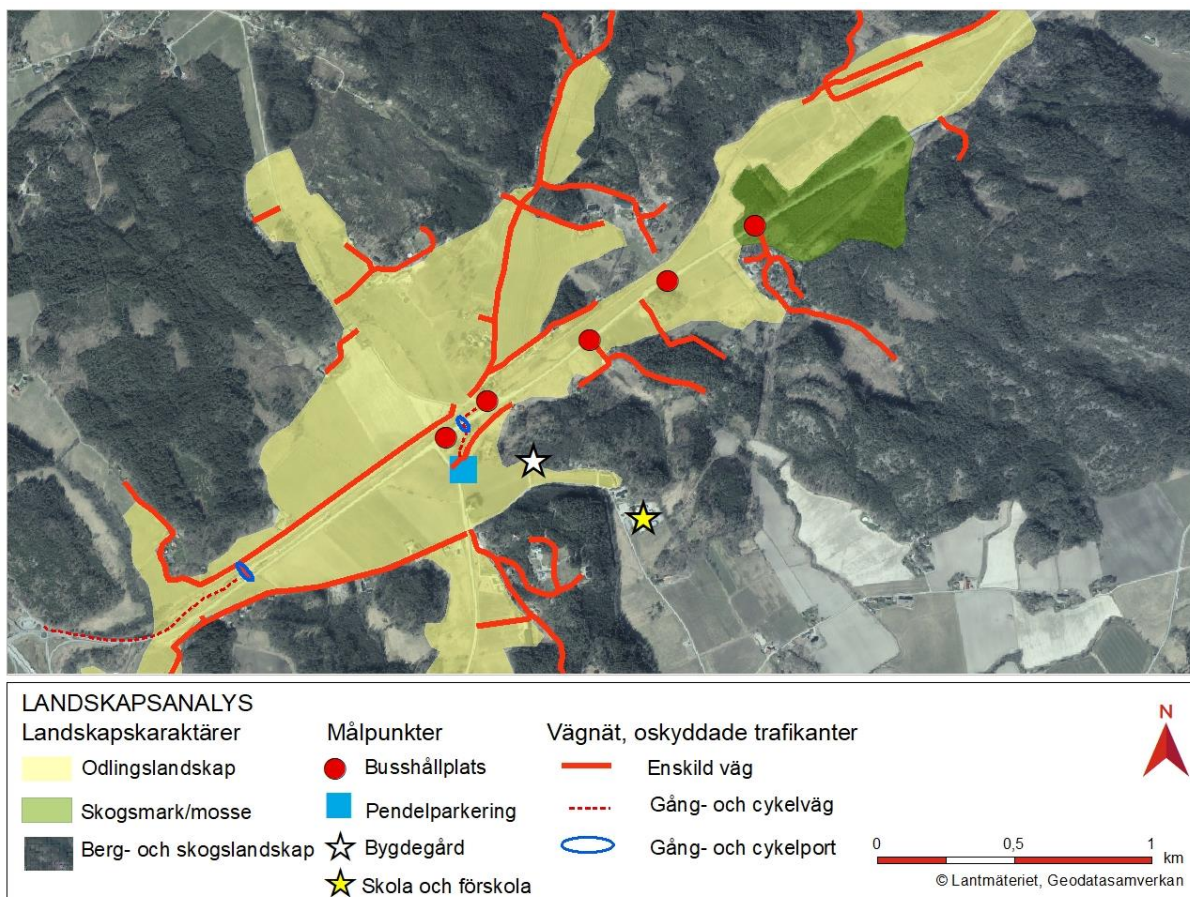
Figur 8. Landskapsanalys.
