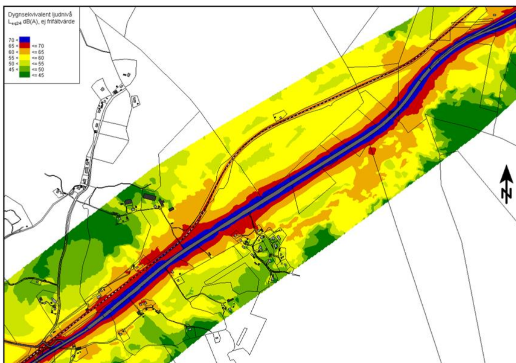
Figur 33. Bullerutbredningskarta som visar utbyggnadsalternativet och dygnsekvivalent ljudnivå i dB(A) för sammanvägd ljudnivå från väg- och spårtrafik. Kartan visar ljudnivån på höjden två meter över mark.
