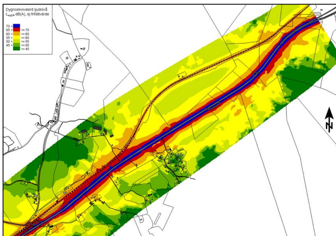
Figur 25. Bullerkarta som visar nollalternativets dygnsekvivalenta ljudnivå i dB(A), sammanvägs ljudnivå från väg- och spårtrafik. Kartan visar ljudnivå två meter över mark.
